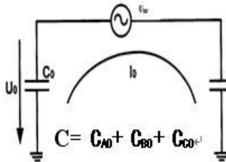
图 3 中性点接 C0 后的等效电路图
