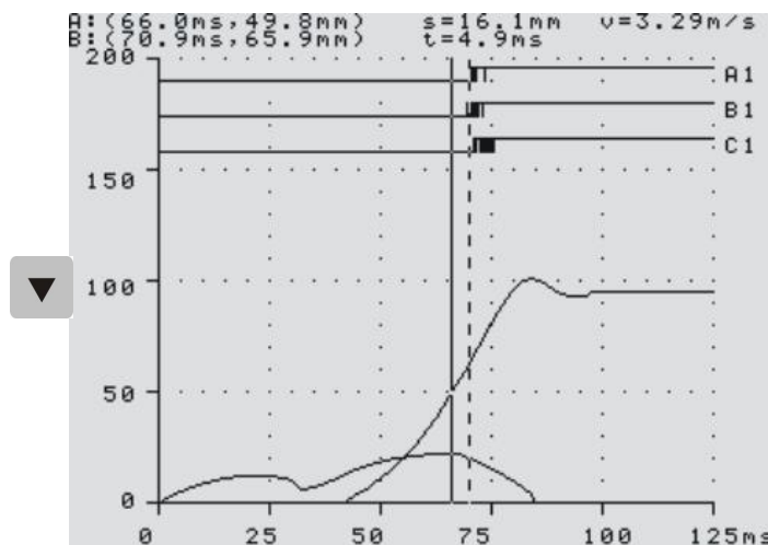
图 6 时间-行程数据曲线图
