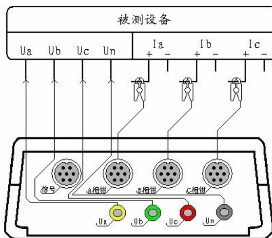
不平衡度测试接线图
