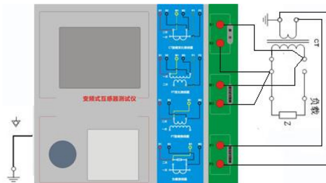
图 2.1 CT 直阻、励磁、变比试验接线方式
