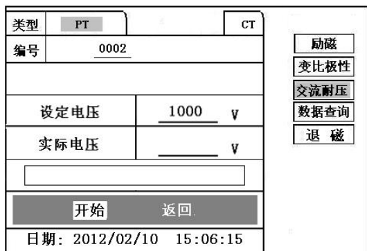
图 23, PT 交流耐压测试界面
