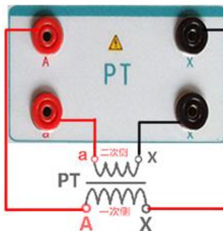
图 22 ，PT 变比极性接线图
