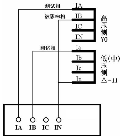
Δ 侧相位调整，按单相短路接线 Ia' = Ia - Ic Ib' = Ib - Ia Ic' = Ic - Ib Y0 侧零序修正，Y 侧的测试相与被影响相相间短路接线
