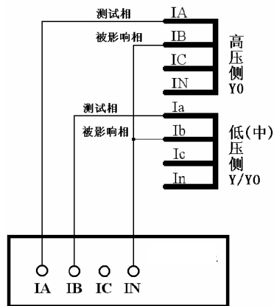
两侧均无相位调整，但有零序修正 两侧均将测试相与零序修正相接成相间短路方式
