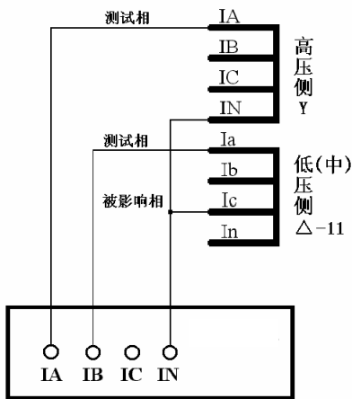
Y 侧相位调整，无零序修正，按单相短路接线 Ia' = Ia - Ib Ib' = Ib - Ic Ic' = Ic - Ia Δ 侧的测试相与被影响相相间短路接线
