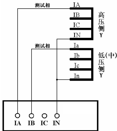
两侧均有相位调整，但无零序修正 两侧均接成单相短路方式
