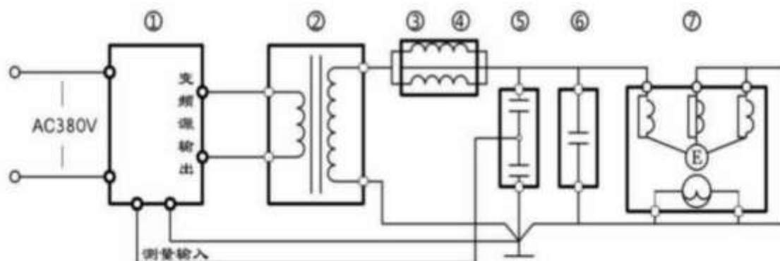
发电机耐压试验接线图
