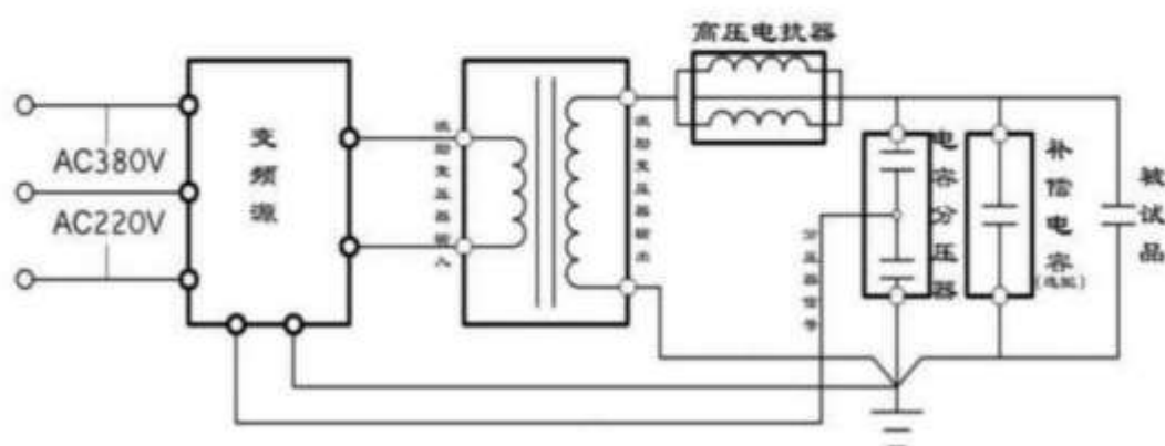
变频串联谐振试验接线图
