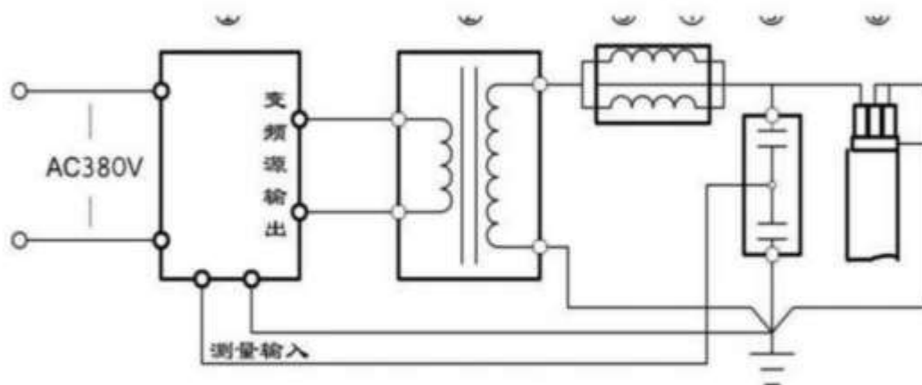
电缆耐压试验接线图
