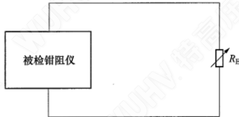
图 4 钳表法测试仪示值误差试验接线图
