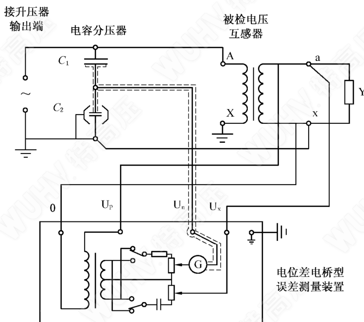
(a) 使用电位差电桥型误差测量装置的检定线路
