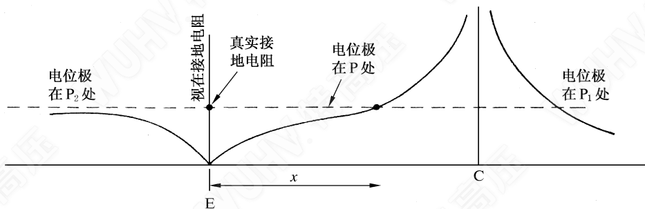
图 7 各种间距 x 时的视在接地电阻
