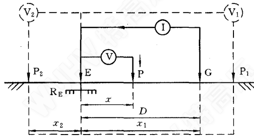
图 C1 电位降法
