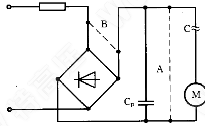
串联电路
