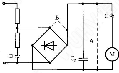
并联电路
