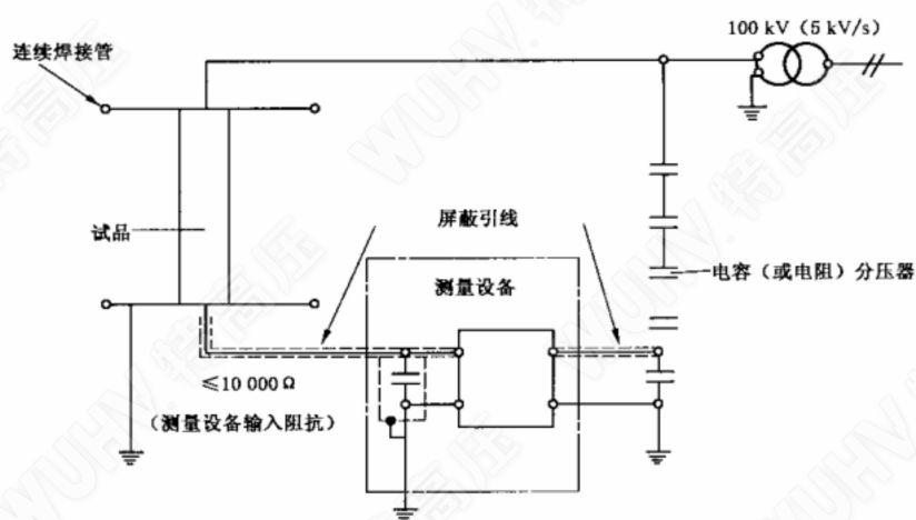
图 A.1 典型试验回路
