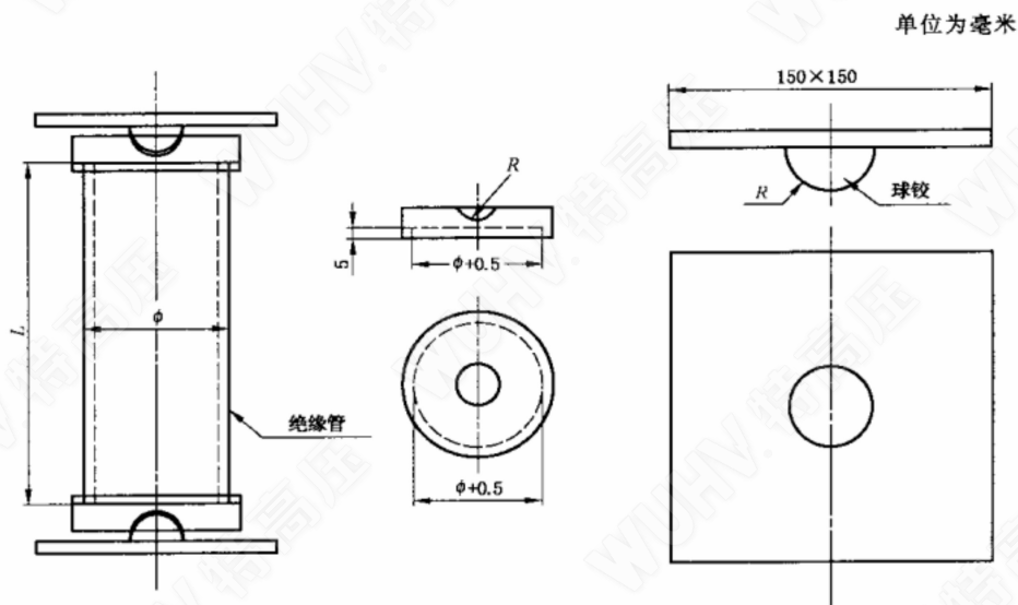
图 C.5 轴向压力试验——绝缘管固定示例
