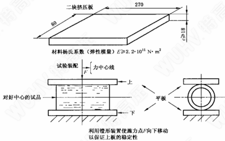
图 C.4 径向挤压试验
