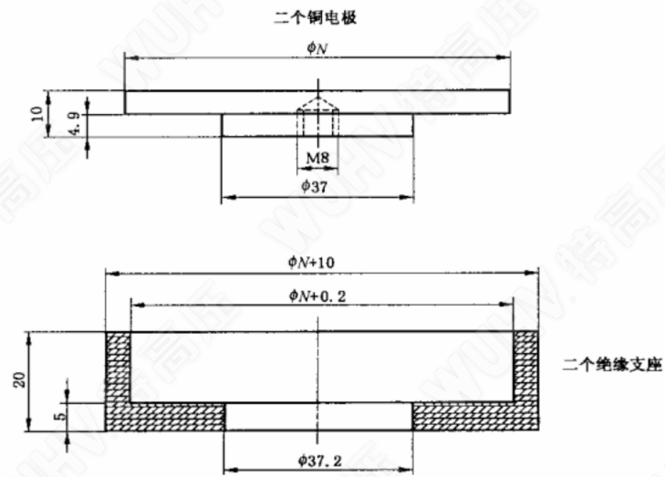
图 A.5 按试样直径配备的保证电极部件结构图
