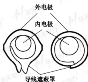
f) 软质导线耐压试验外电极
