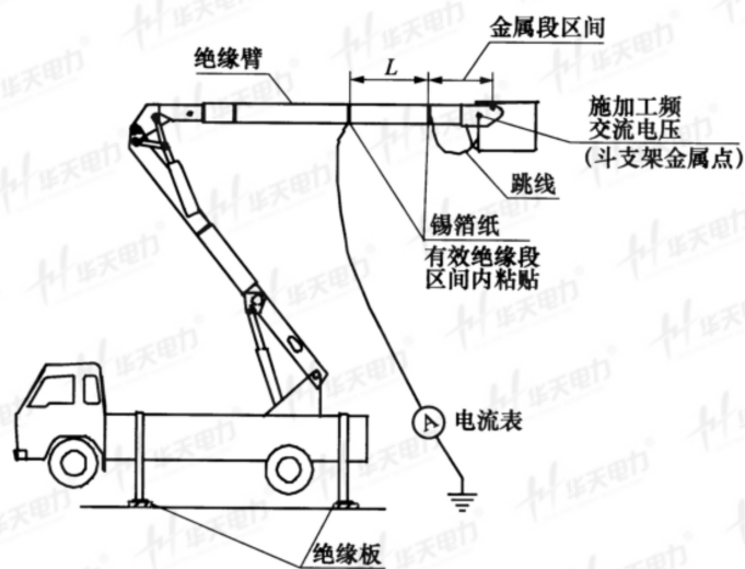
b) 折叠臂式和混合式斗臂车交流耐压试验布置
