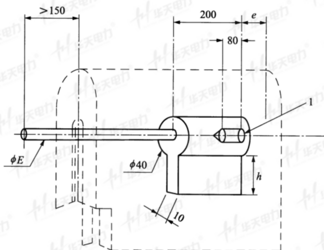
b) 耐张装置遮蔽罩的电极
