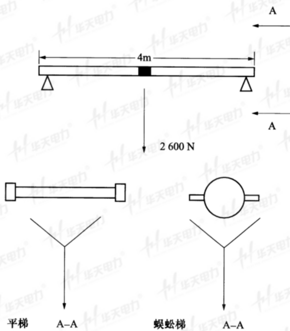
a) 水平强度试验布置
