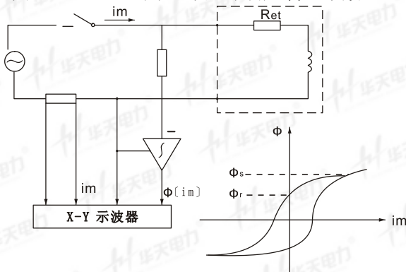
图 E. 0. 2-2 用磁滞回环确定剩磁系数 K。
