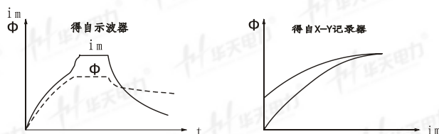
图 E. 0. 2-4 典型记录曲线
