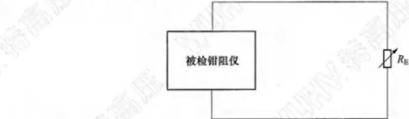
图 4 钳表法测试仪示值误差试验接线图
