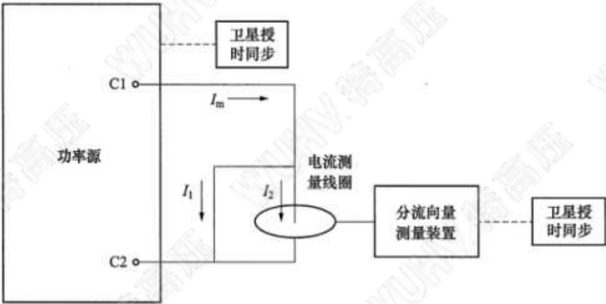
图 A.2 非主从模式工作原理
