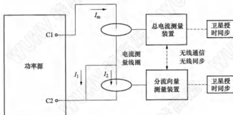
图 A.1 主从模式工作原理
