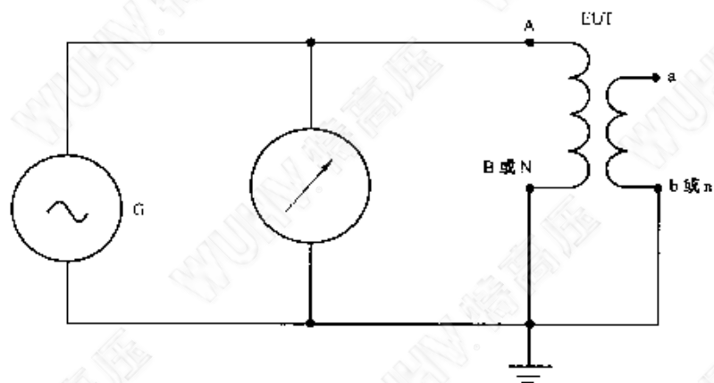
图 311 外施工频耐压试验的试验电压应用
