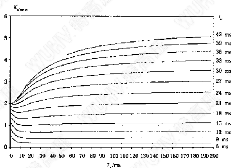
图 2E.6 K_d 的确定(在时间范围 1 及 16.7 Hz 和 T_s = 5.5 s 条件下)
