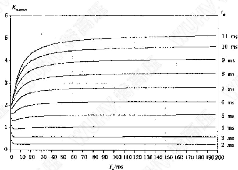
图 2E.4 K_d 的确定(在时间范围 1 及 50 Hz 和 T_s = 1.8 s 条件下)
