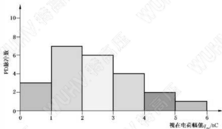
b) 在以下视在电荷 q_m 范围内出现的局部放电脉冲数 m : 0 nC~1 nC, 1 nC~2 nC, 2 nC~3 nC, 3 nC~4 nC, 4 nC~5 nC
