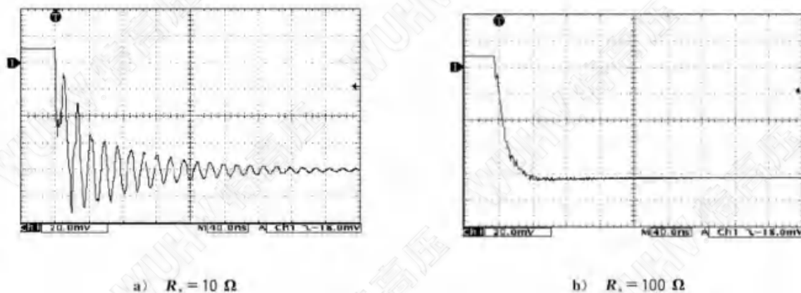
图 B.4 串联电阻 R_s 对采用图 B.3 所示回路的 C_m 上出现的阶跃电压响应的影响, 其中示波器通过一段长 1 m 和 50 \Omega 测量电缆连接到校准器
