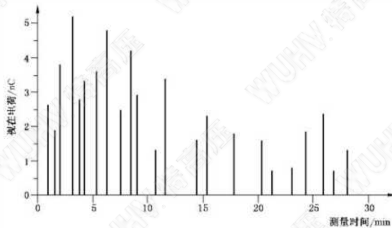
a) 单个局部放电脉冲的视在电荷
