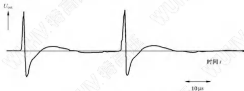
a) 带宽 \Delta f = 45 \text{ kHz} \sim 440 \text{ kHz} , 短时输入脉冲
