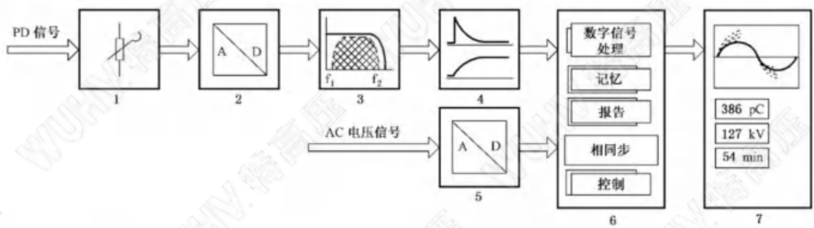
图 F.2 配有电子积分器的模拟局部放电仪的框图
