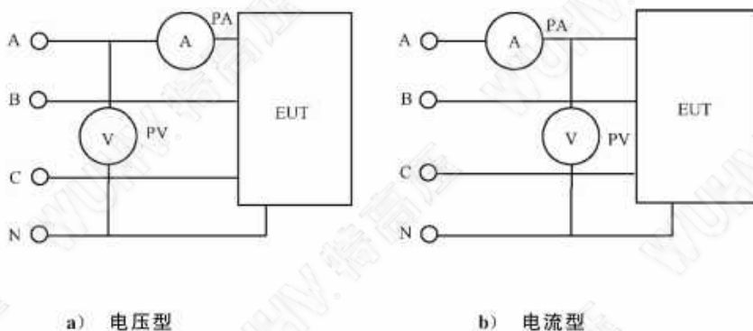
图 24 三相四线对称输入电路示例
