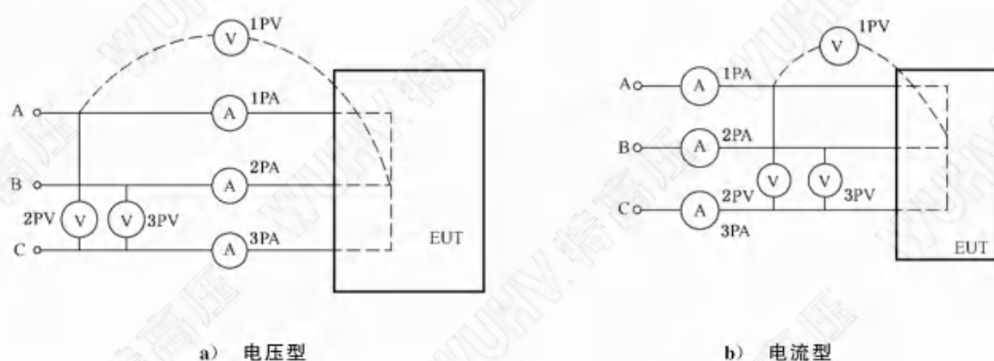
图 26 三相三线输入电路示例
