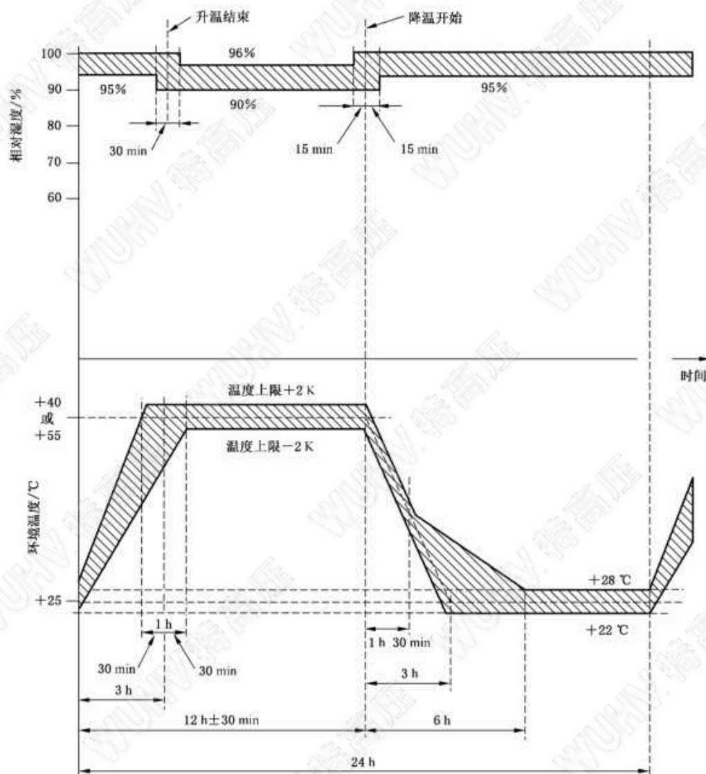
图 29 交变湿热循环方法一
