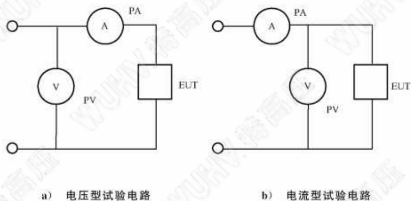
图 23 单输入激励量试验电路示例
