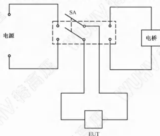
图 27 线圈直流电阻测试电路示例
