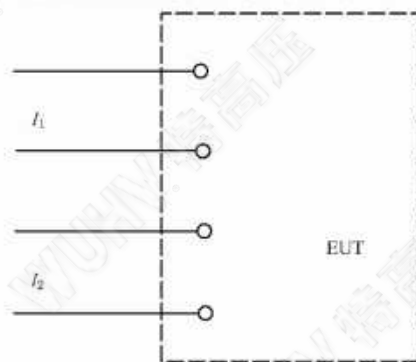
图 17 两个电流激励量的试验电路示例
