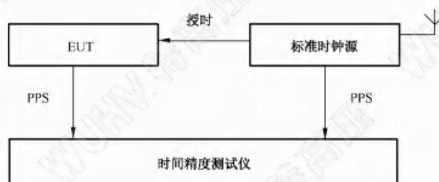
图 21 PPS 秒脉冲比对法试验接线示意图
