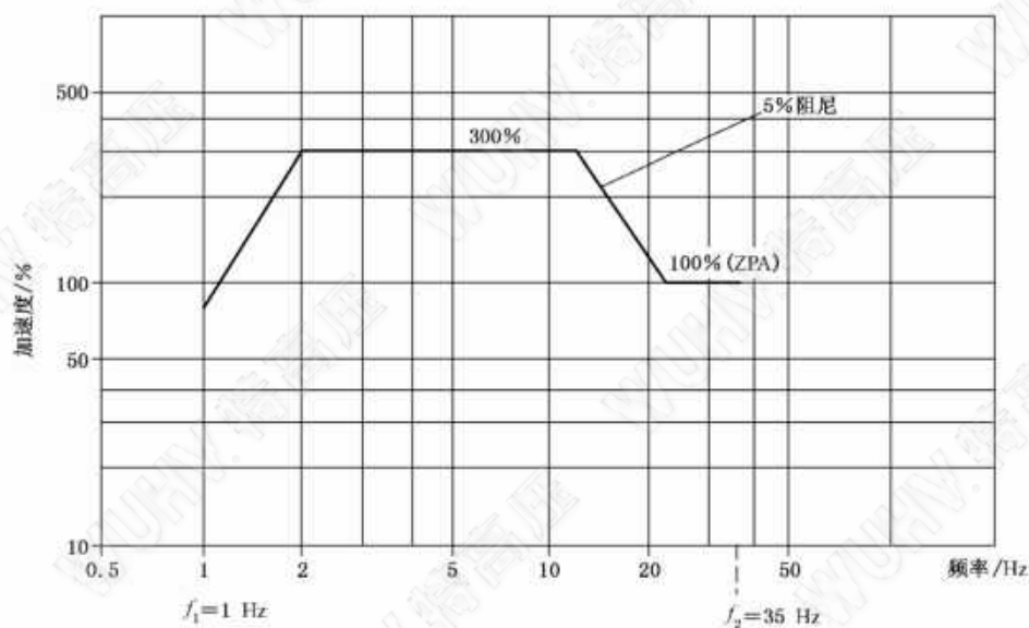
图 32 多频宽带标准响应谱形状
