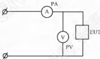
图 37 保护联结阻抗试验电路示例
