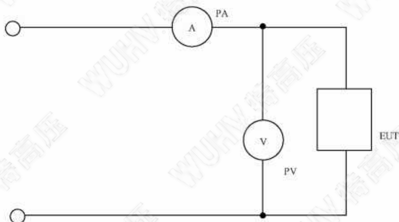
图 5 电压型线圈电阻测量电路示例
