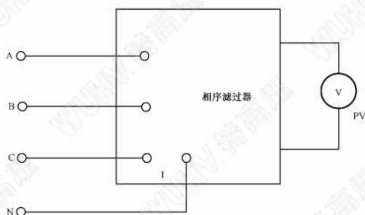
图 11 相序过滤器输出电压测试电路示例
