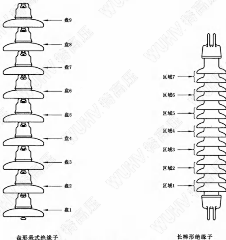
图 C.1 测量 ESDD 和 NSDD 用绝缘子串
