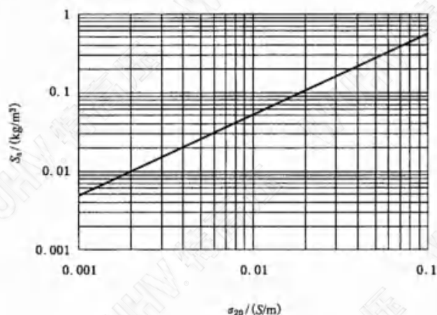
图 C.4 \sigma_{20} 和 S_s 的关系
