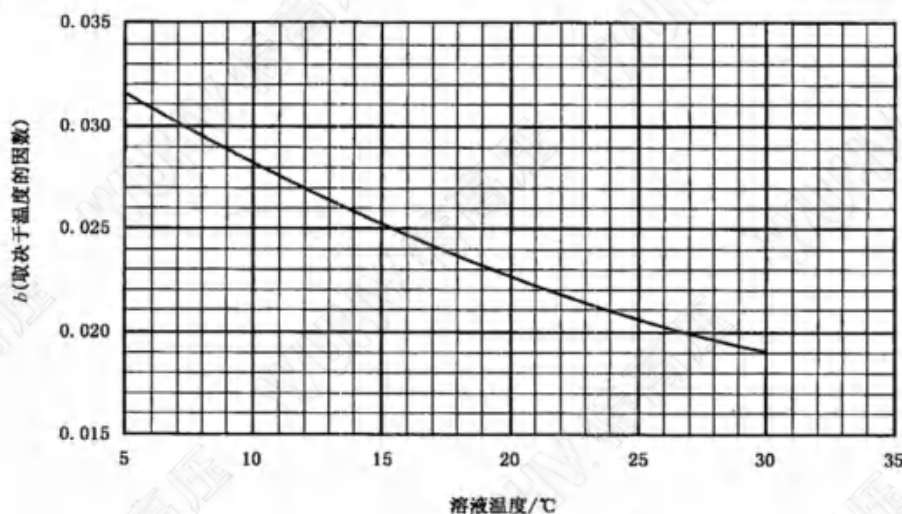
图 C.3 b 值
