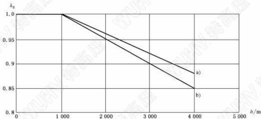
图 3 温升的海拔校正因数
