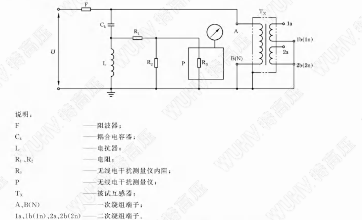
图 4 无线电干扰电压试验线路
