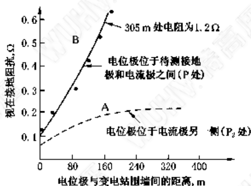
图 9 低阻抗接地系统实例
