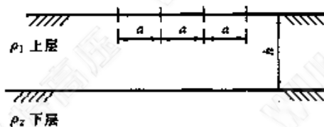
图 A1 两层土壤
