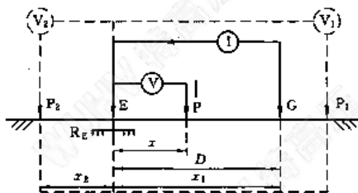
图 C1 电位降法
