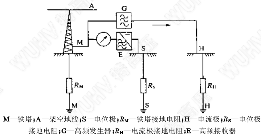
图 19 高频土壤电阻仪
