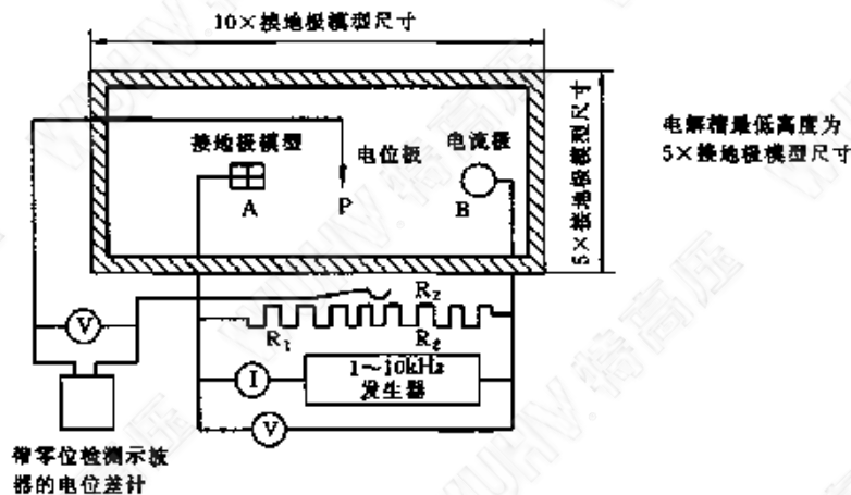
图 13 电解槽
