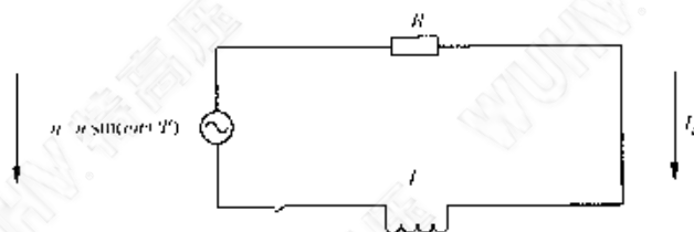
图 G.1 短路试验的等效电路图
