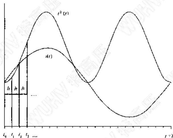
图 G.3 瞬时电流的真有效值和瞬时电流的平方值的数值估算方法
