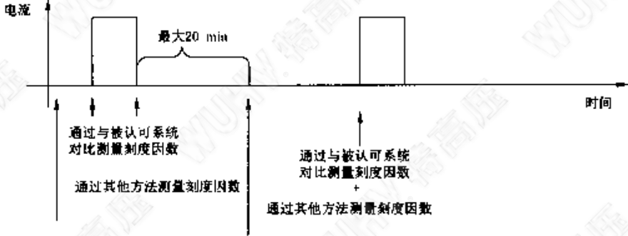
图 7 脉冲电流和短时电流的短时稳定性试验
