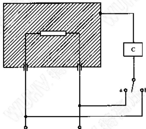
图1 单相连接的Ⅱ类器具在工作温度下泄漏电流的测量电路图
