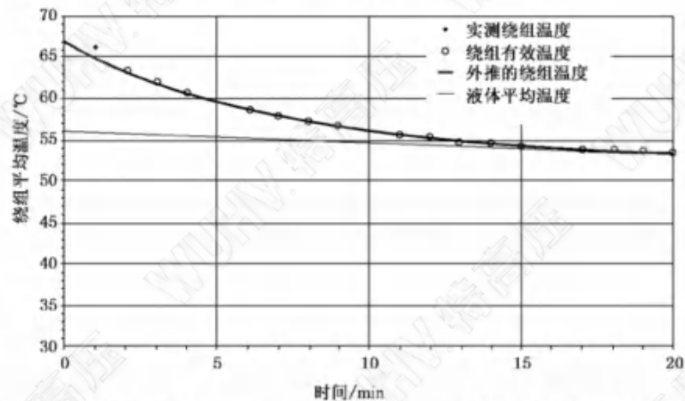
图 B.4 用拟合曲线 \theta_{\text{w}}(t) = A_0 - kt + g \times e^{-t/T_{\text{w}}} 外推出的冷却曲线
