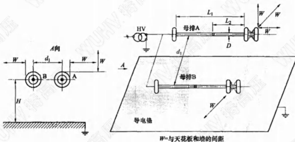
图 5 试验布置图
