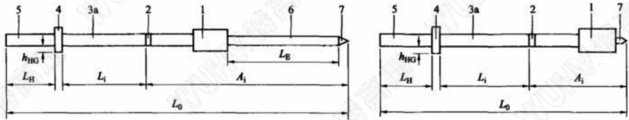
a) 有接触电极延长段的整体式验电器
