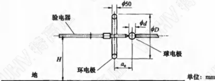
图 3 球电极在环电极之后的试验布置
