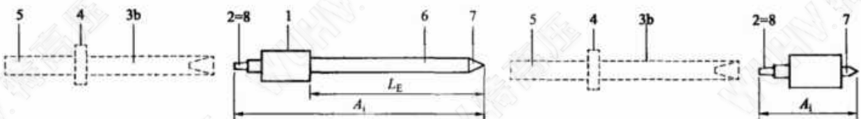
a) 有接触电极延长段的分体式验电器
