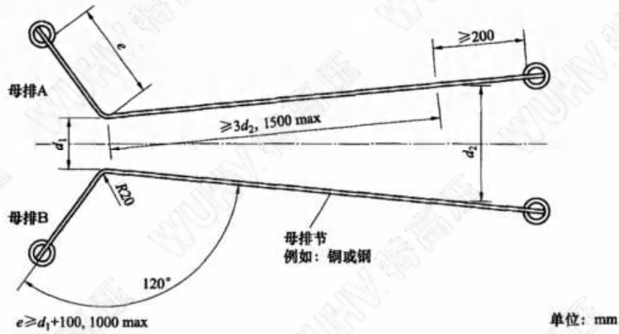
图 17 试验布置和 V 形母排的尺寸
