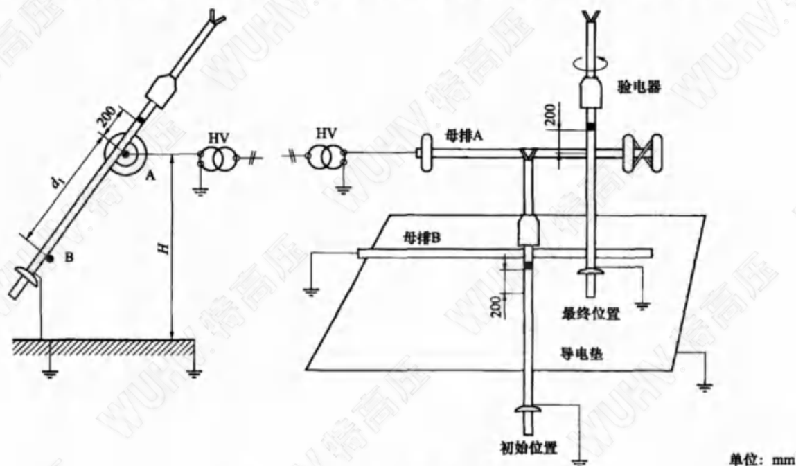
图 21 平行母线电极布置的沿面耐压试验
