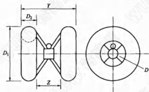
图7 双屏蔽环的尺寸(导电材料)
