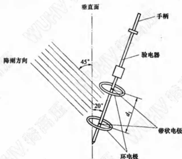
图 23 户外型验电器防短接试验
