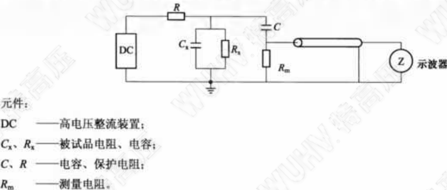
图 2 用示波器测量纹波
