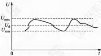
图 1 纹波波形
