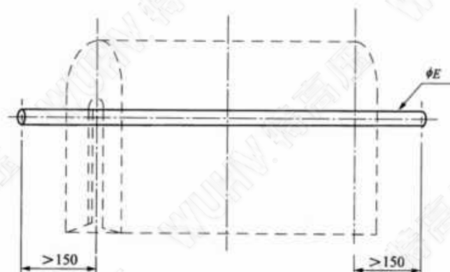
a) 硬质导线遮蔽罩电极
