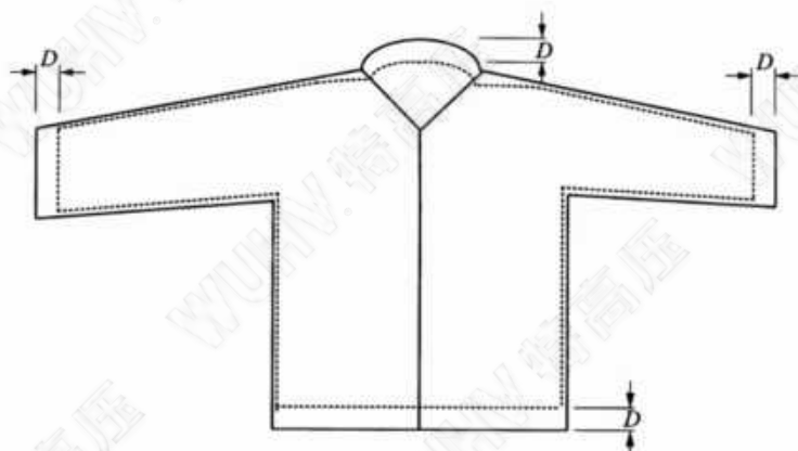
b) 绝缘上衣内电极布置示意图
