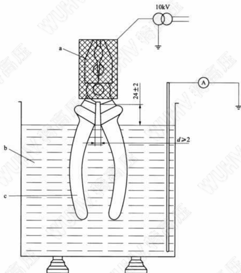
a) 包覆绝缘工具电气试验装置
