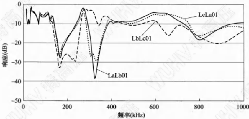
a) 变形时
