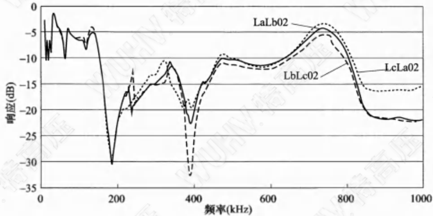
b) 修复后
