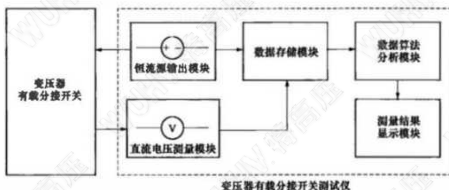
图1 测试仪恒流输出工作原理框图
