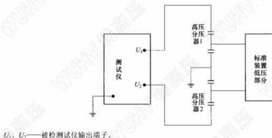
图 3 电压测量误差试验接线图
