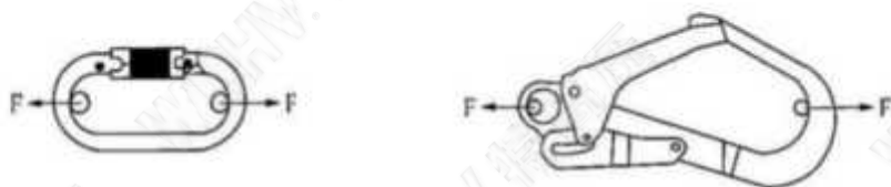
图C.5 连接器静负荷试验示意图
