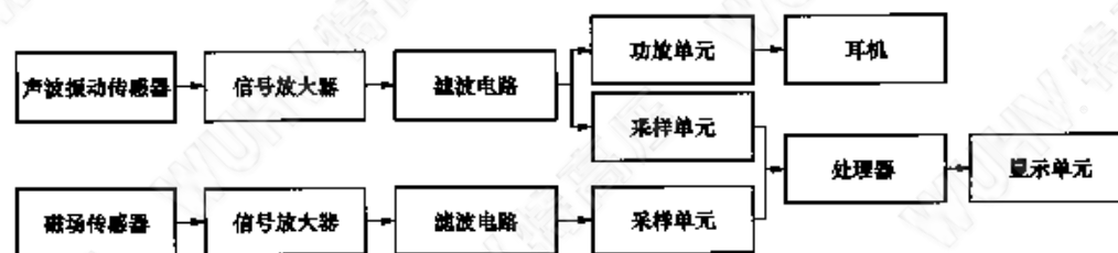
图 2 采用声磁同步法的定点仪原理框图
