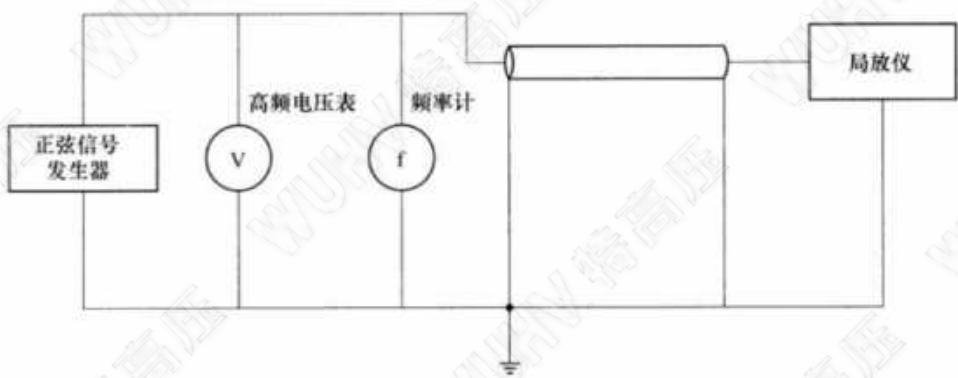
图 1 频带与截止频率试验接线图
