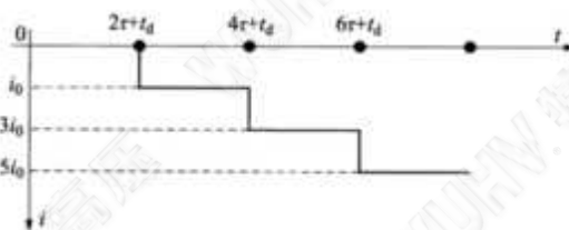
图 B.9 测量端电流幅值图
