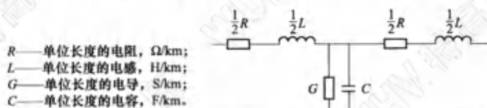
图 A.1 一小段电缆的等效电路
