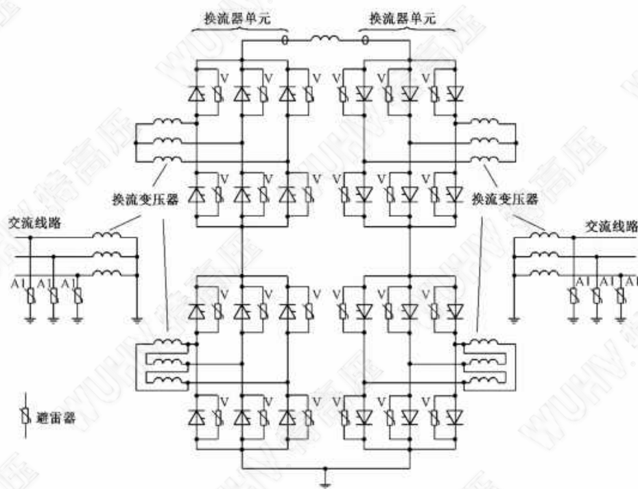
图 18 高压直流换流站避雷器保护方案示例
