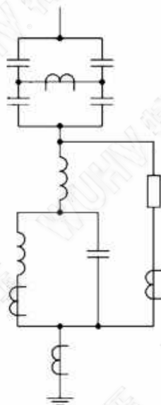
图 5 滤波器有限接地故障保护示例
