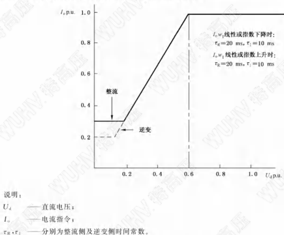
图 2 低压限流特性示例
