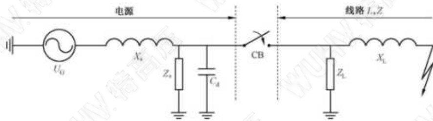
图 48 符合 7.109.3 的近区故障试验的基本回路布置和 b1) 类预期 TRV 回路:电源侧有 ITRV 和线路侧有时延 (续)
