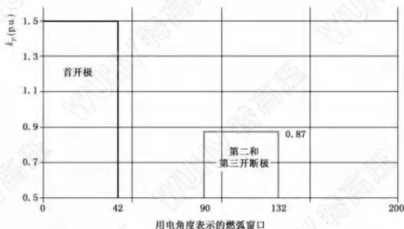
图 40 对于 k_{pe} 为 1.5 的系统, 燃弧窗口和决定各极 TRV 的电压系数 k_p 的图形表示
