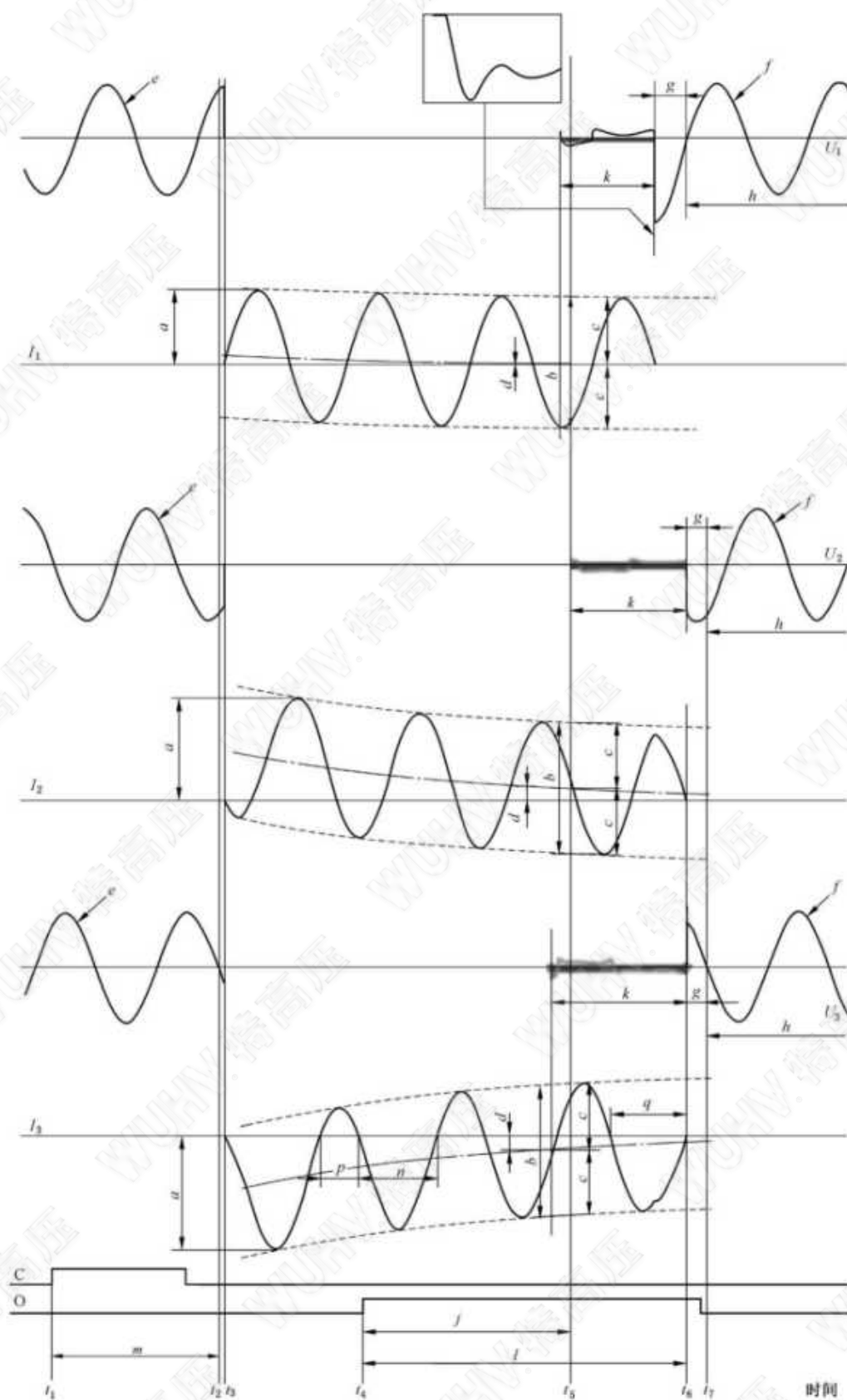
图1 三相短路关合—开断循环的典型波形图
