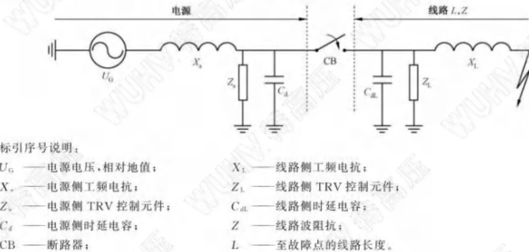
图 47 符合 7.109.3 的近区故障试验的基本回路布置和 a) 类预期 TRV 回路：电源侧和线路侧均有时延
