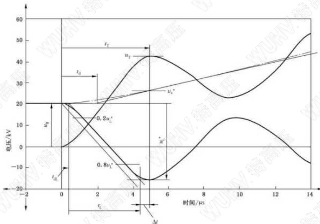
图 1.1 线路侧和电源侧 TRV 参数的典型图示—线路侧和电源侧均有时延
