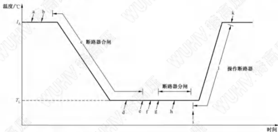
图 11 低温试验试验顺序
