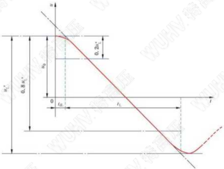
图 50 有时延的线路侧瞬态恢复电压的示例
