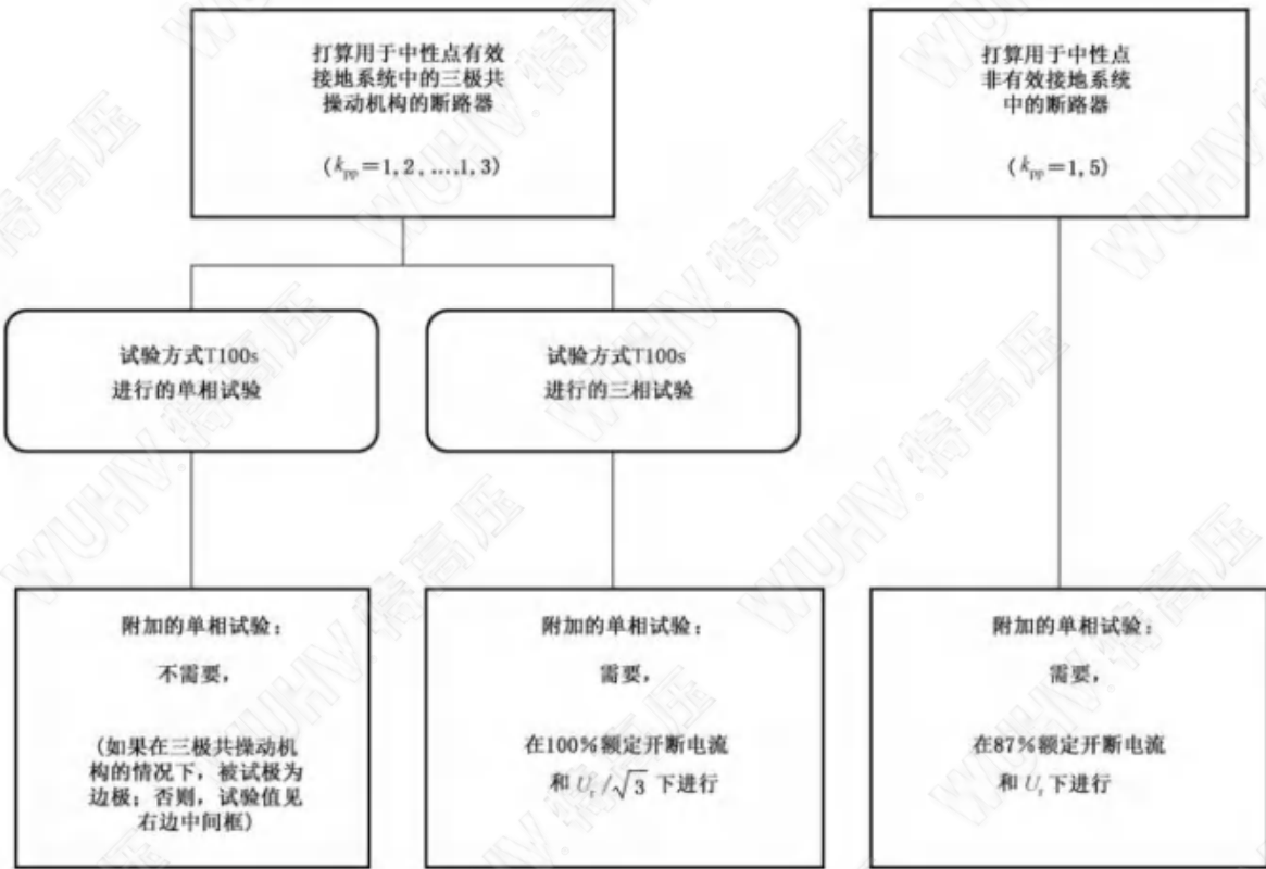
图 46 附加的单相试验的必要性和试验要求
