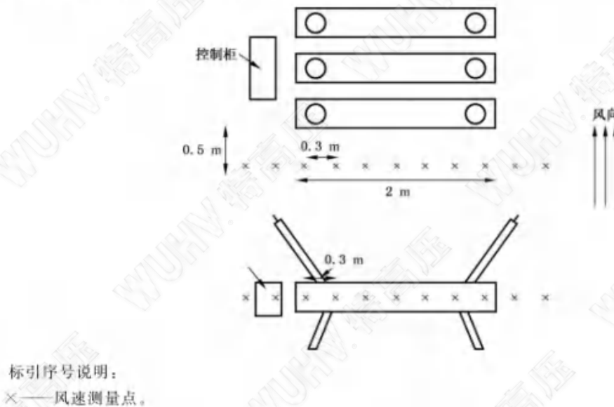
图 10 风速测量示例
