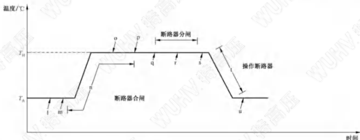
图 12 高温试验试验顺序
