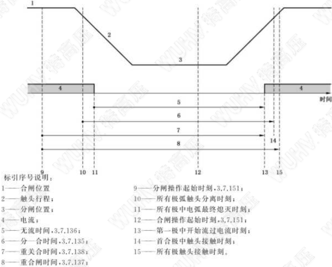
图4 不带分合闸电阻器的断路器的重合闸(自动重合闸)
