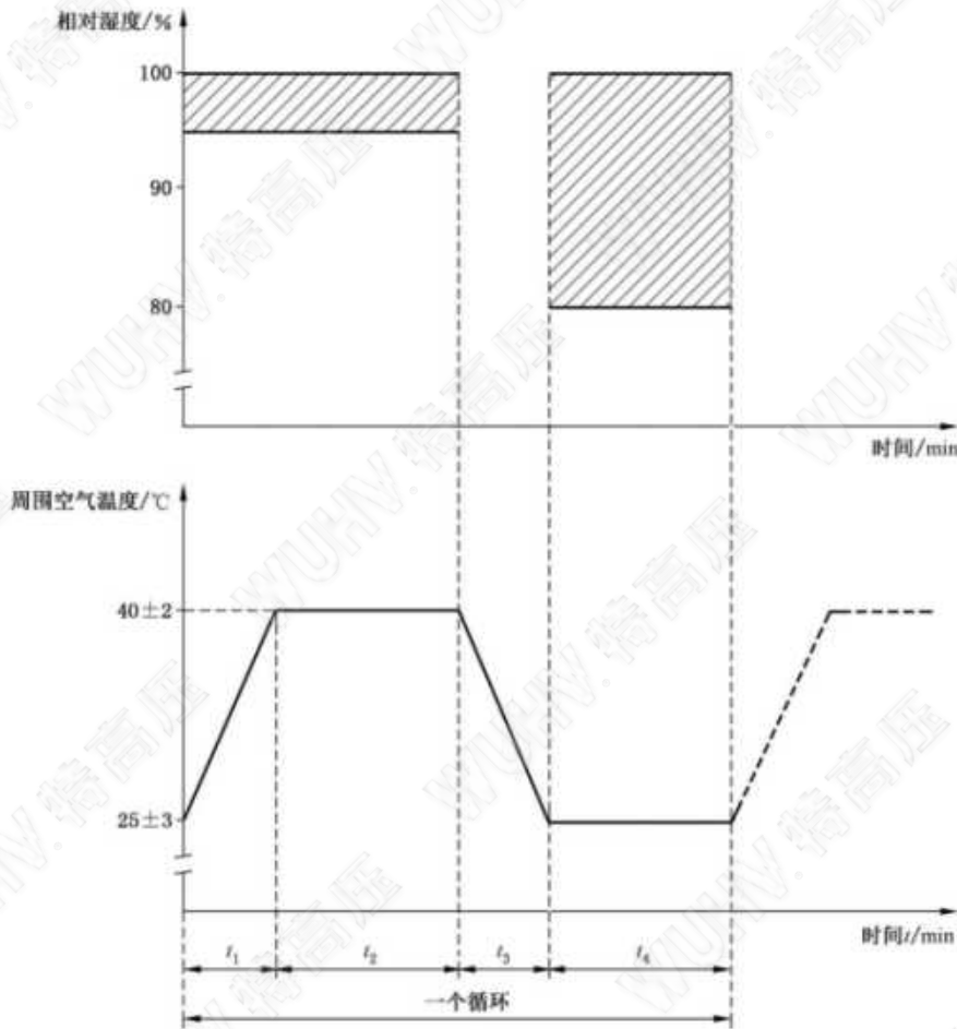
图 13 湿度试验
