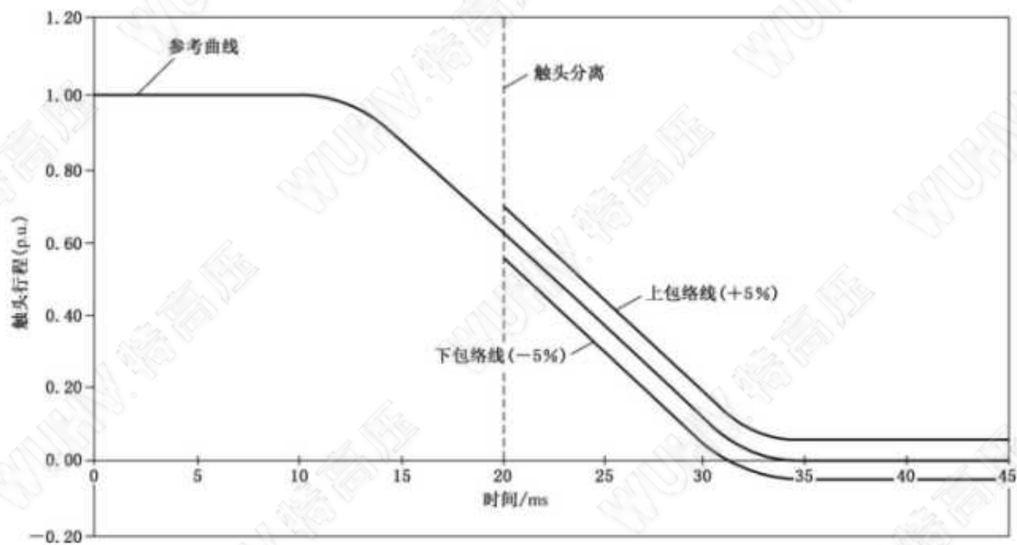
图 15 图 14 中的参考机械行程特性曲线及其以参考曲线为中心的包络线 (+5%, -5%)
