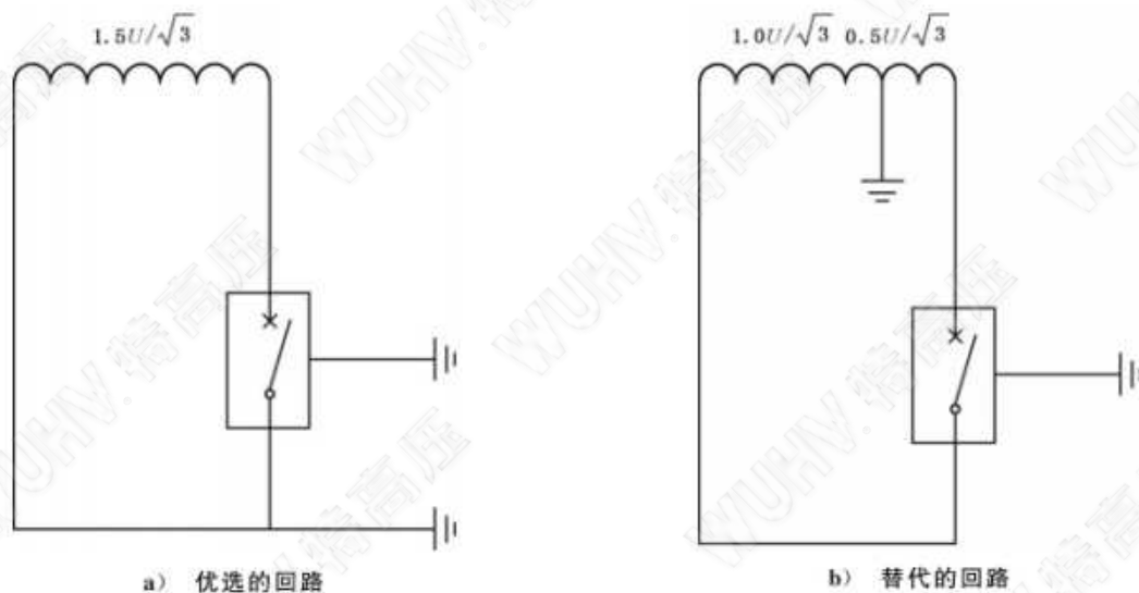
图 19 k_{sp} = 1.5 ，单相短路试验的试验回路的接地
