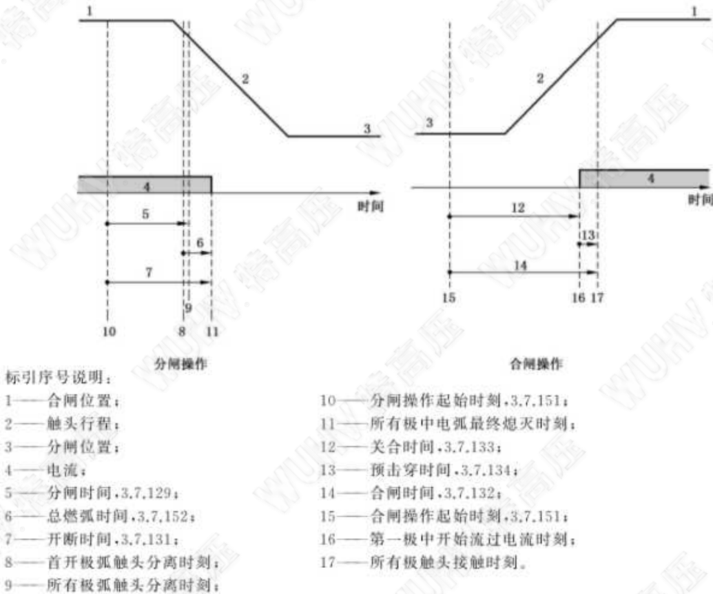
图 2 不带分合闸电阻器的断路器的分闸和合闸操作
