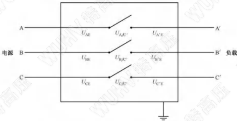
图 D.1 表 D.1、表 D.2 和表 D.3 中考虑的试验布置
