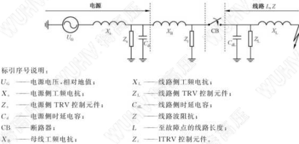
图 48 符合 7.109.3 的近区故障试验的基本回路布置和 b1) 类预期 TRV 回路: 电源侧有 ITRV 和线路侧有时延
