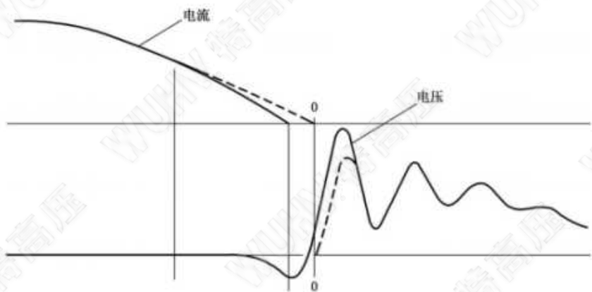
图 G.2 存在电弧电压时的开断
