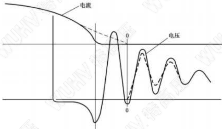
图 G.3 理想开断时的 TRV
