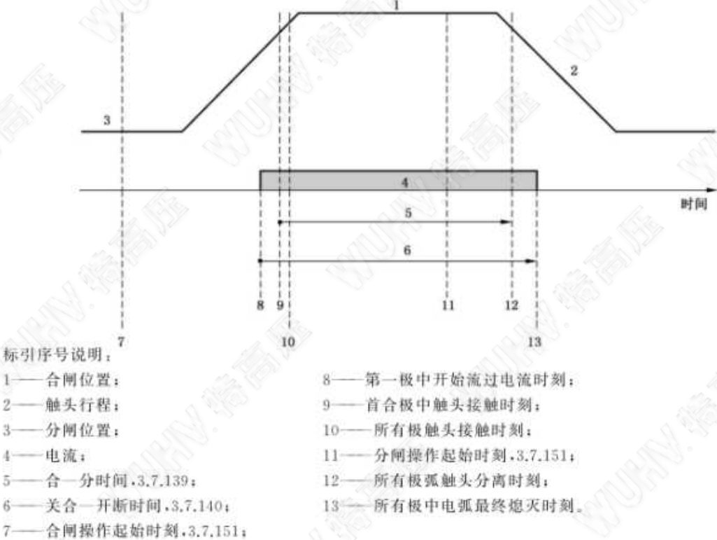
图3 不带分合闸电阻器的断路器的合一分循环
