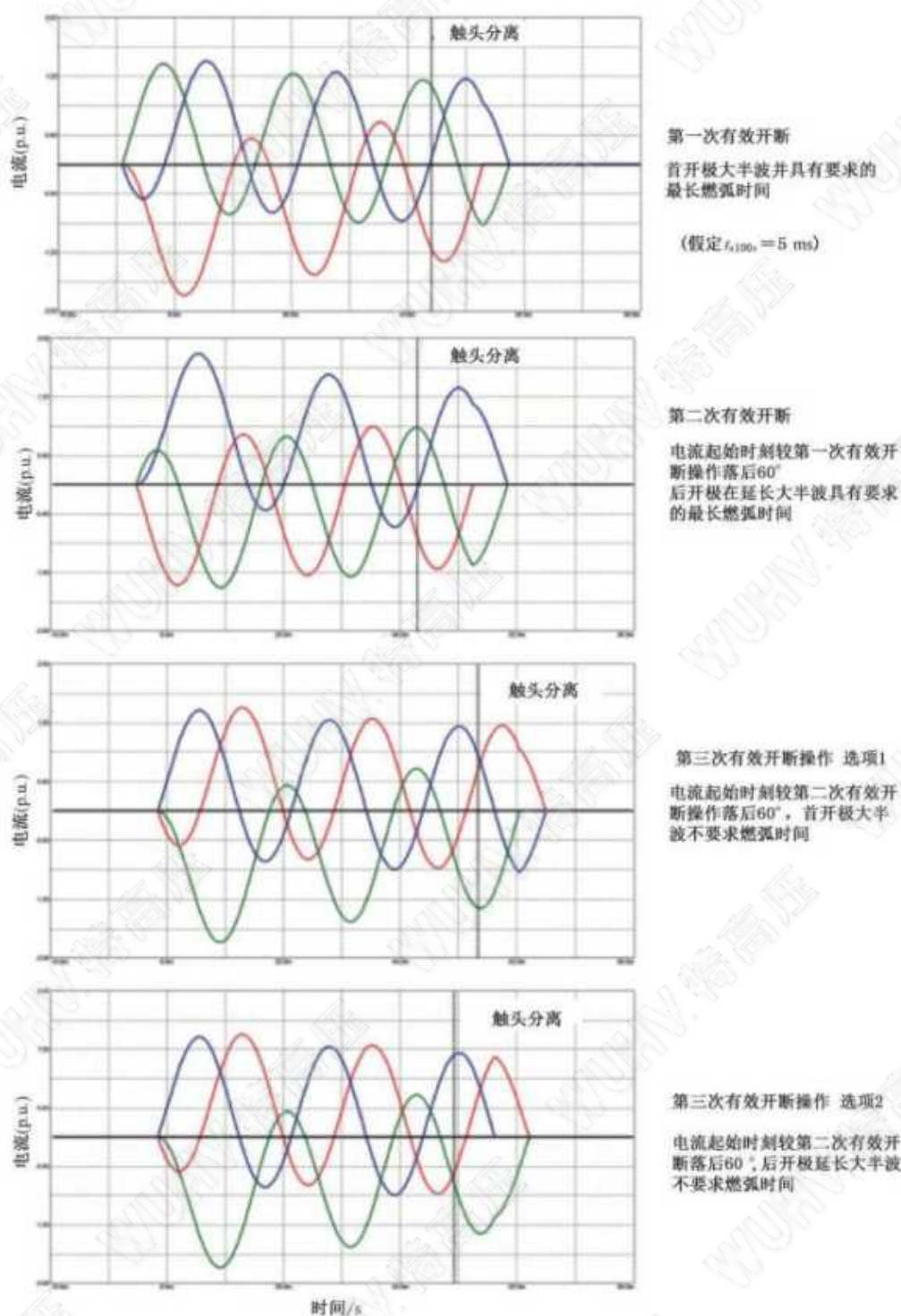
图 33 k_{pp} = 1.5 , 三相试验时 3 次有效非对称开断操作的图例
