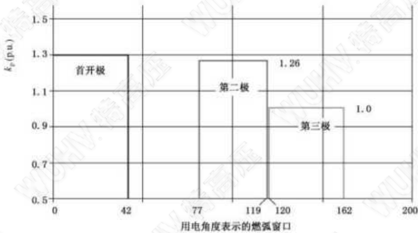
图 39 对于 k_{op} 为 1.3 的系统,燃弧窗口和决定各极 TRV 的电压系数 k_p 的图形表示
