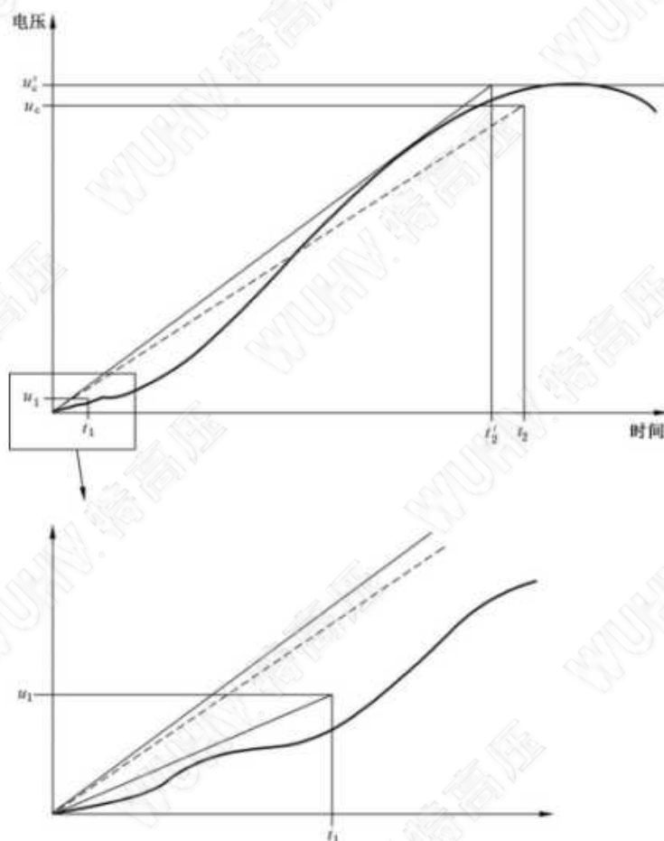
图 53 容性电流开断试验的恢复电压
