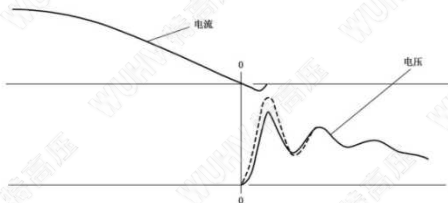
图 G.6 有弧后电流时的开断
