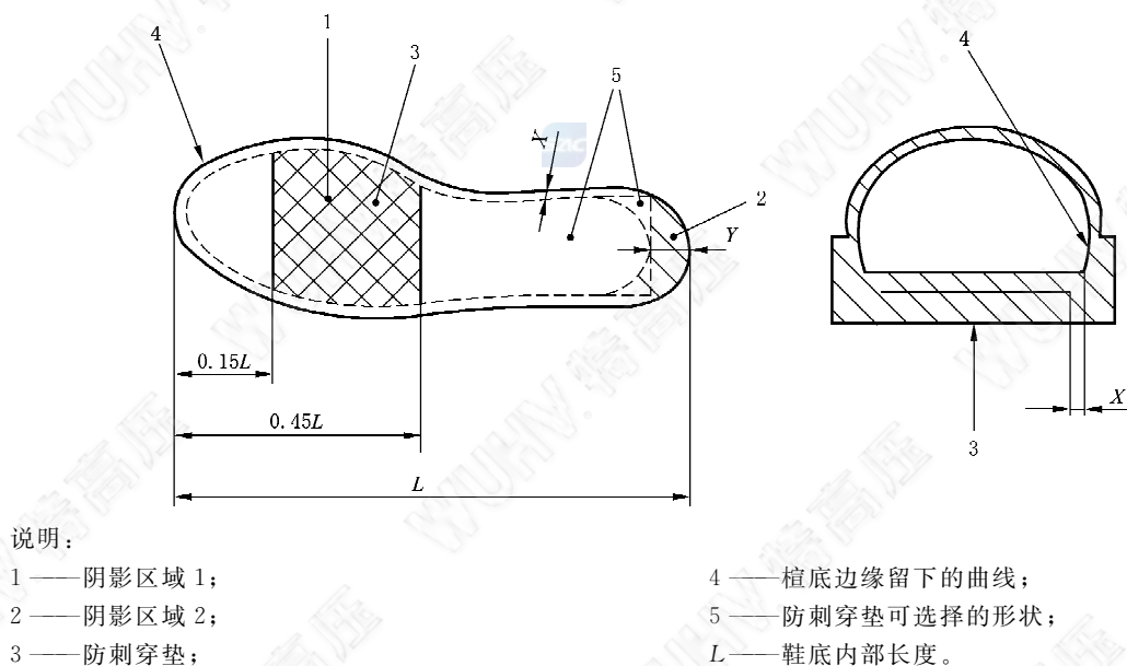
图 10 防刺穿垫的位置
