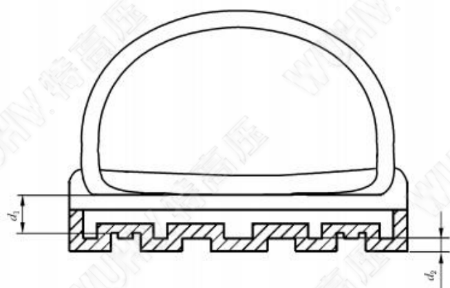
图 6 直接注压、硫化和胶粘的外底
