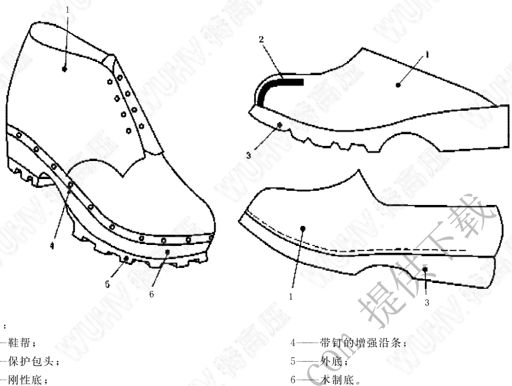
图 2 其他鞋(Ⅰ类)部件示意图
