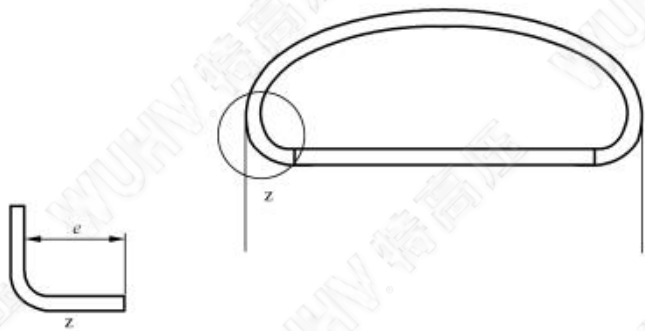
图 9 保护包头卷边宽度 e
