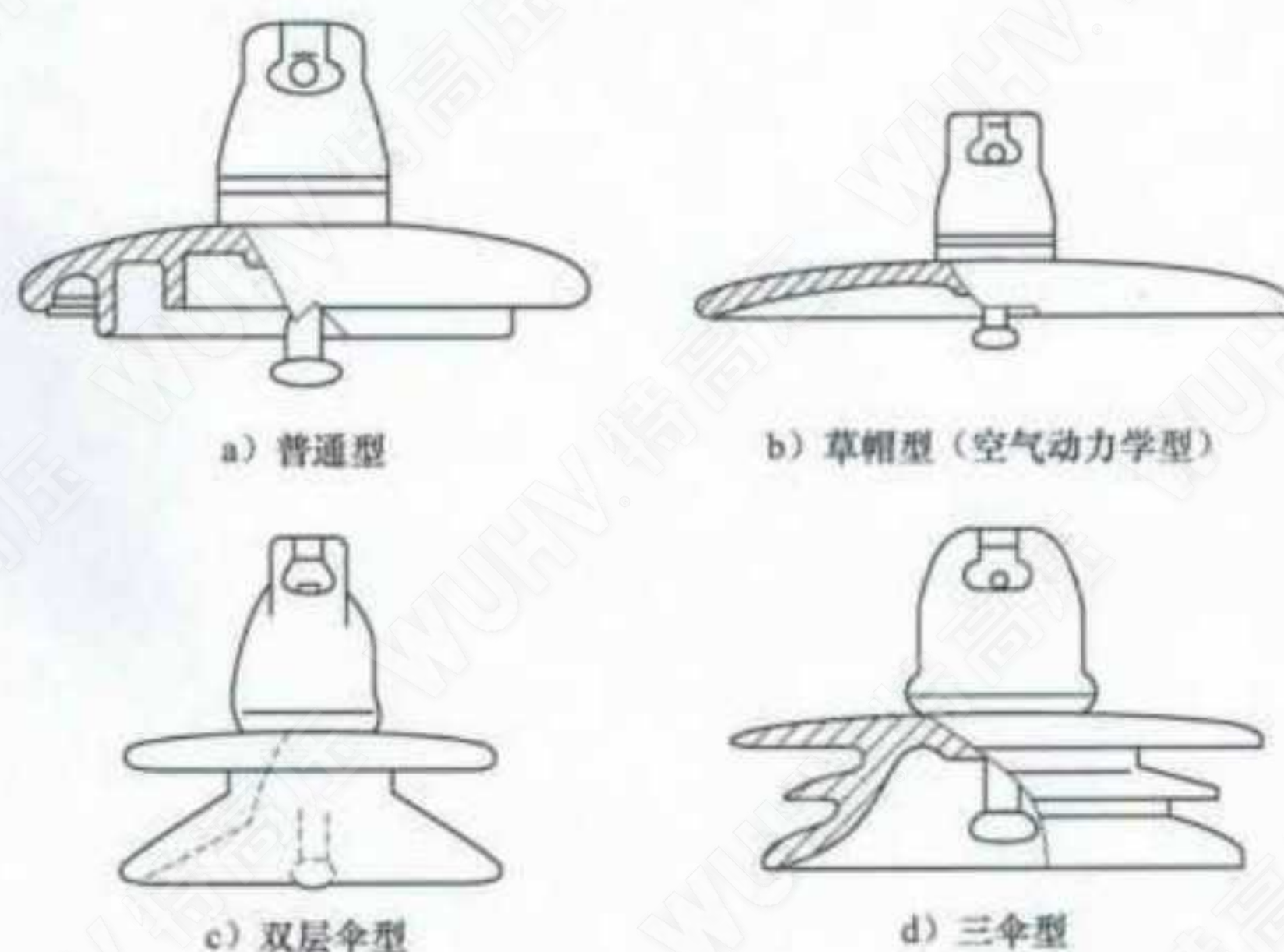
图 D.1 盘形悬式绝缘子的典型外形图
