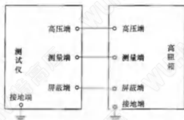
图 8 体积电阻率测量试验接线示意图
