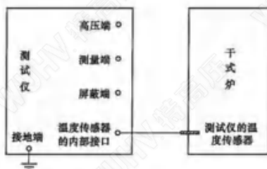
图6 温度测量误差试验接线示意图
