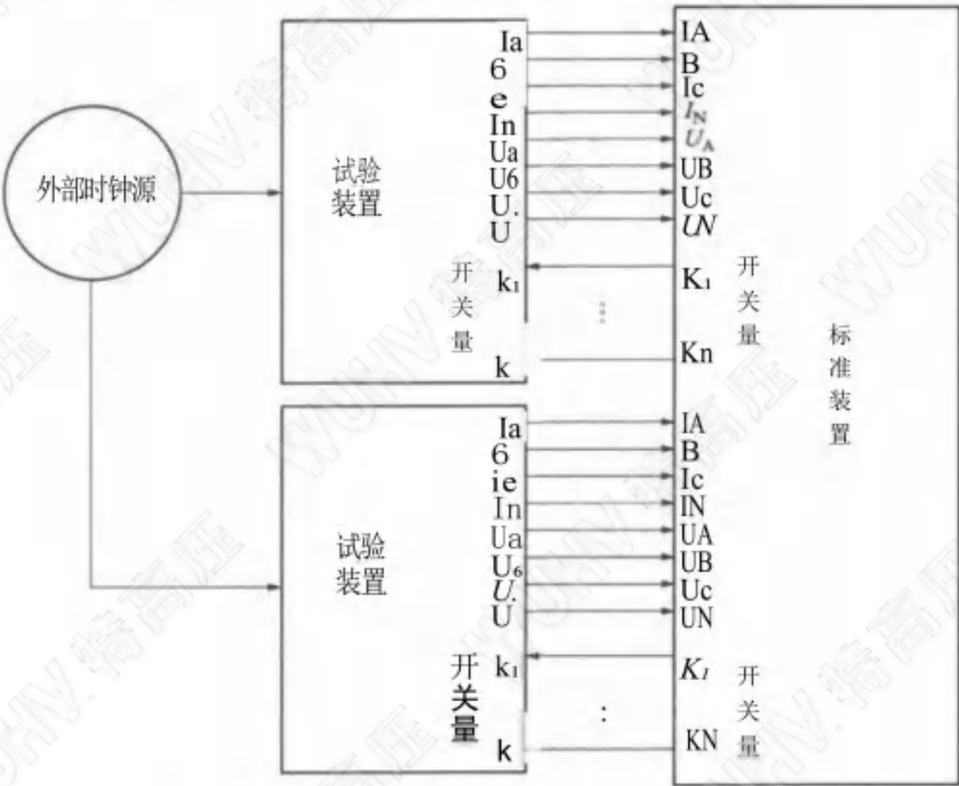
图A.8 试验装置多机输出同步性测试接线图
