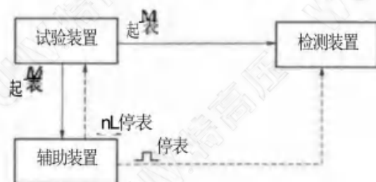
图 A.10 试验装置时间测量能力检测接线图
