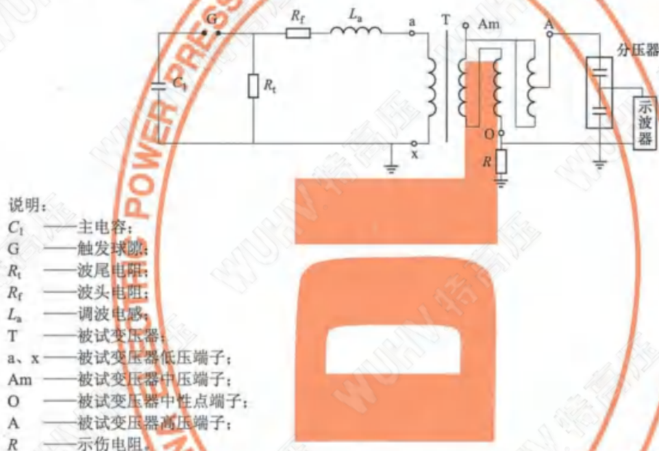
图 B.1 单相自耦变压器振荡操作冲击试验接线示意图
