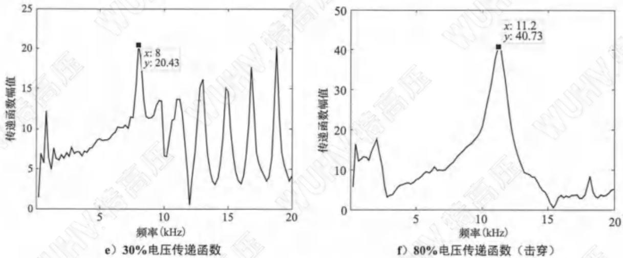
图 D.2 某主变压器振荡操作冲击试验 80%电压内绝缘击穿(续)
