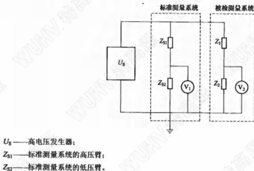
图 3 示值误差接线图
