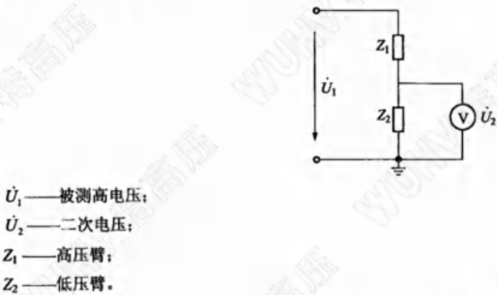
图 1 高电压分压器测量装置原理图
