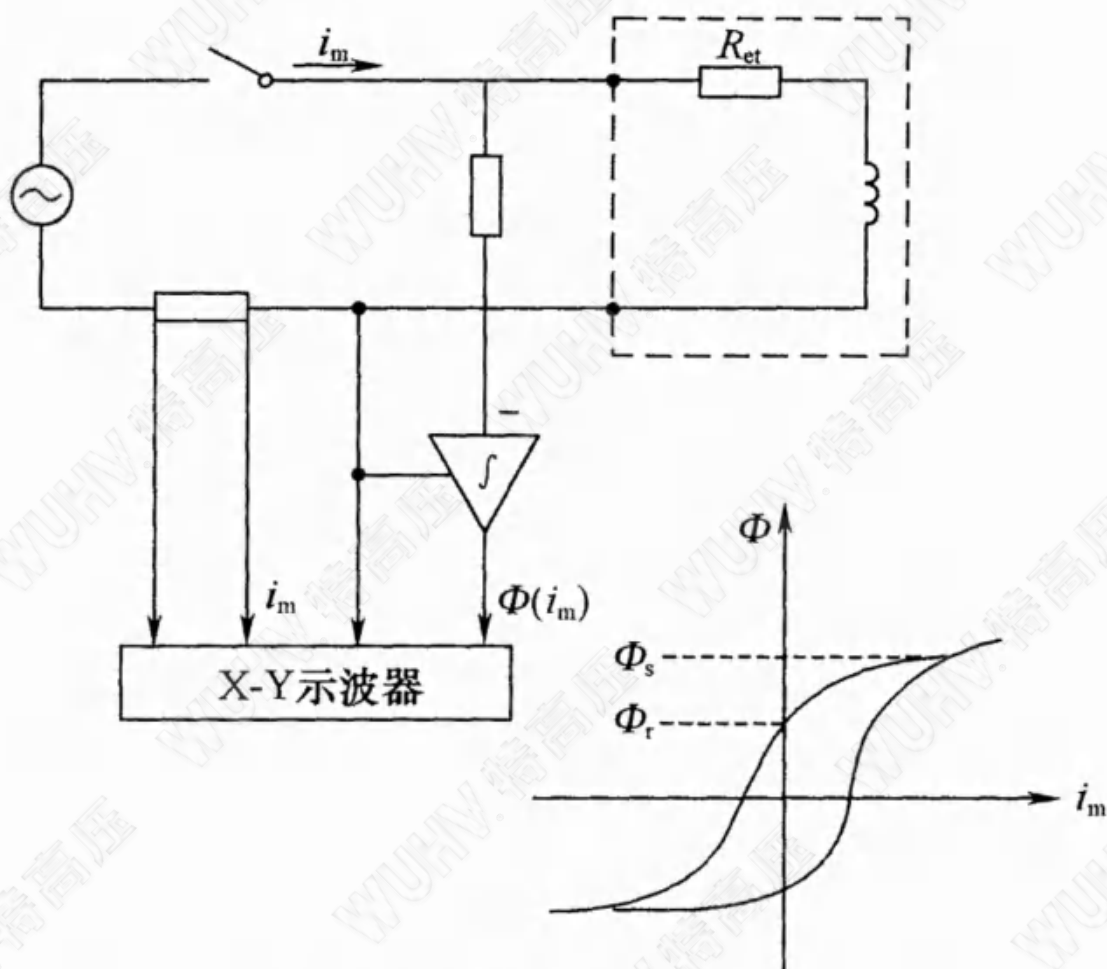
图3 用磁滞回环确定剩磁系数 K_t
