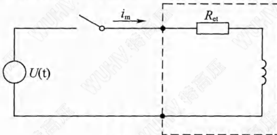
图 2 基本电路
