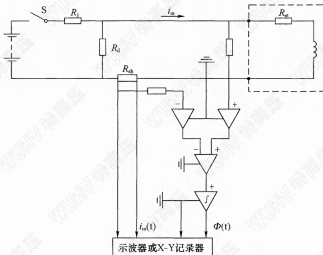
图 4 直流法基本电路
