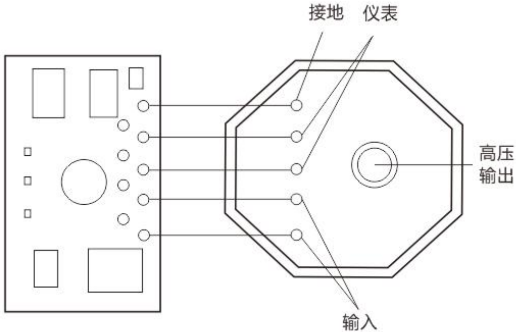
XC系列接线图
