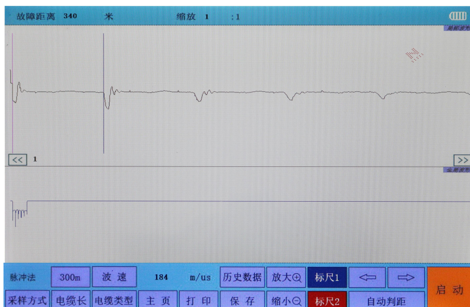
低压脉冲法测量图形
