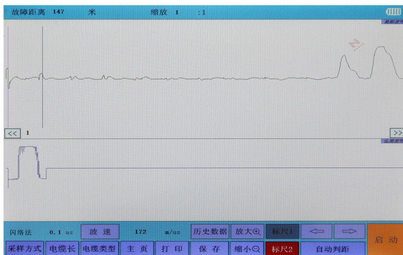
冲击闪络法测试波形示例
