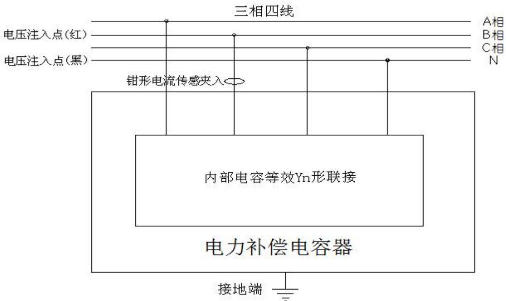
图 29Yn 形联接被试电容 Bn 相接线图
