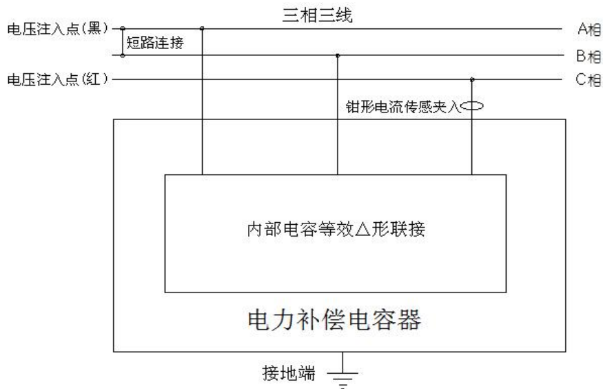
图 24 \Delta 形联接被试电容 CA 相接线图
