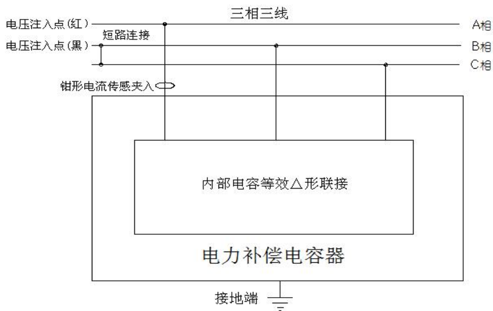
图 22 \Delta 形联接被试电容 AB 相接线图
