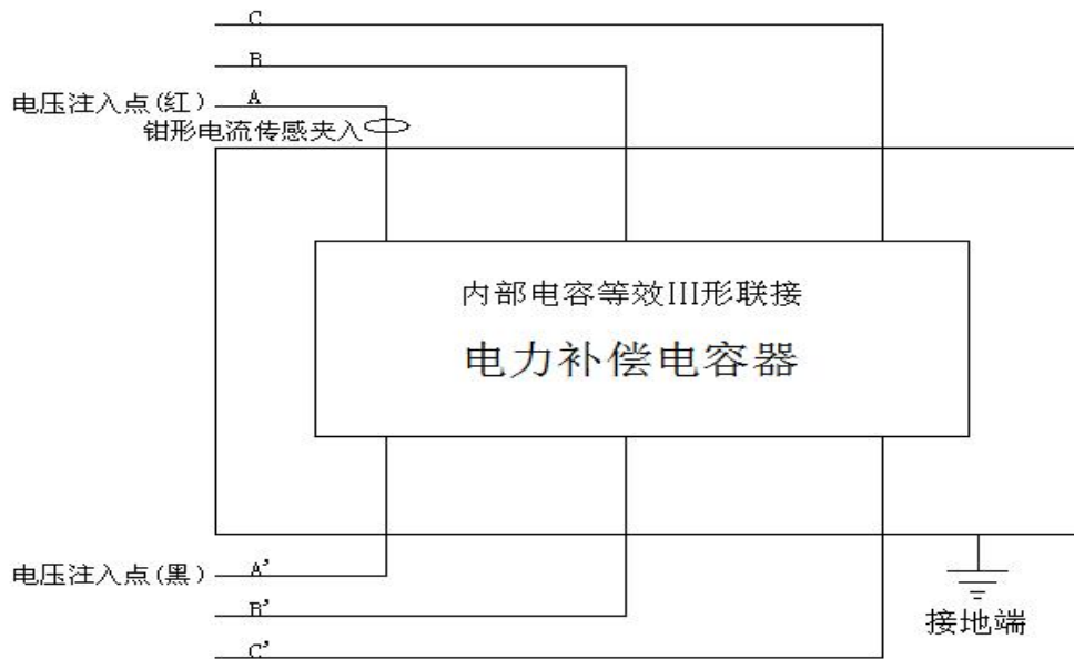
图 31III 形联接被试电容接线图
