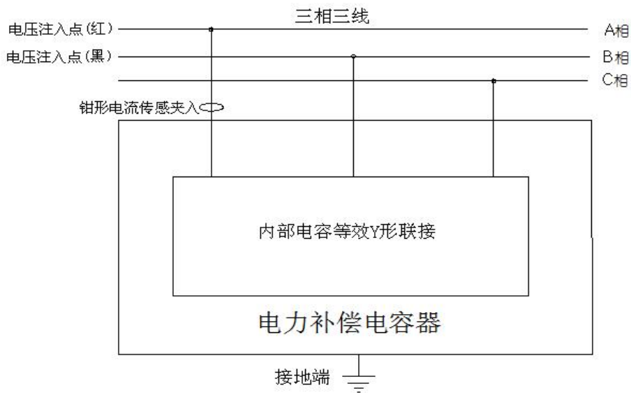
图 25Y 形联接被试电容 AB 相接线图
