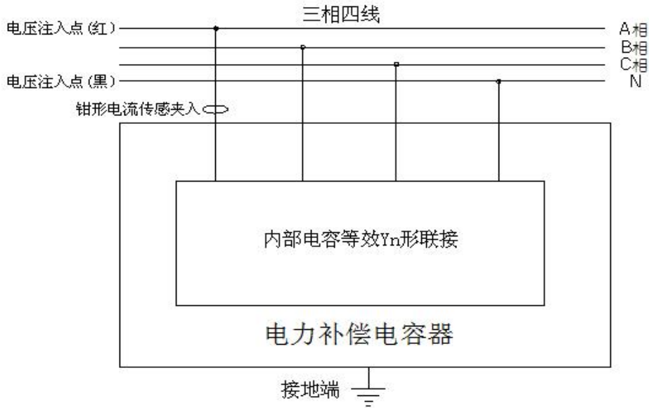
图 28Yn 形联接被试电容 An 相接线图
