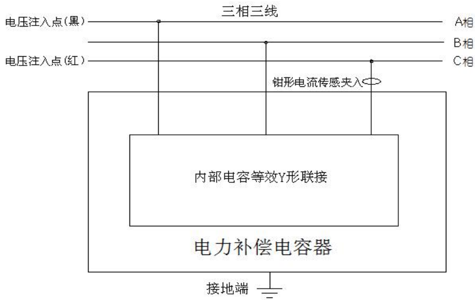
图 27Y 形联接被试电容 CA 相接线图
