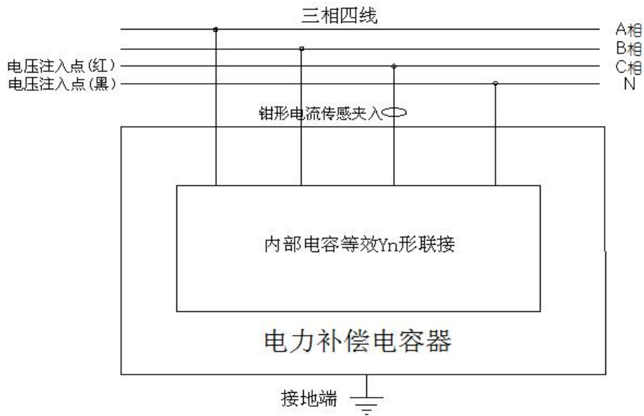
图 30Yn 形联接被试电容 Cn 相接线图
