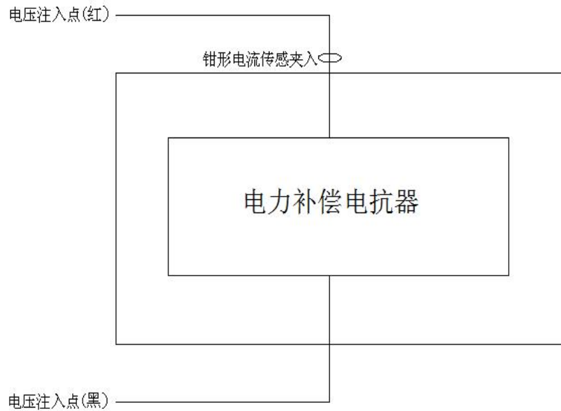
图 32 被试电抗器电感接线图
