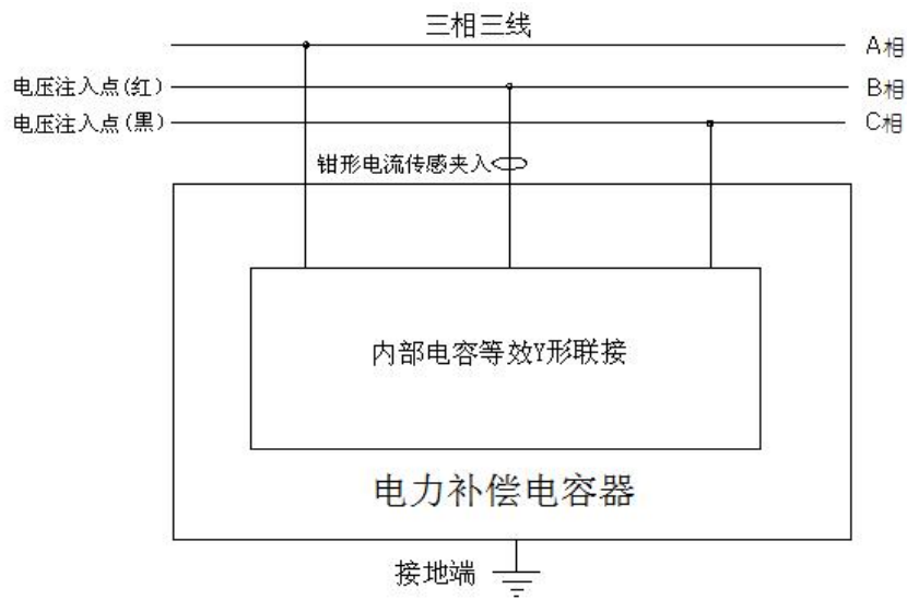
图 26Y 形联接被试电容 BC 相接线图
