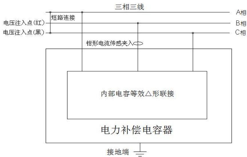
图 23 \Delta 形联接被试电容 BC 相接线图
