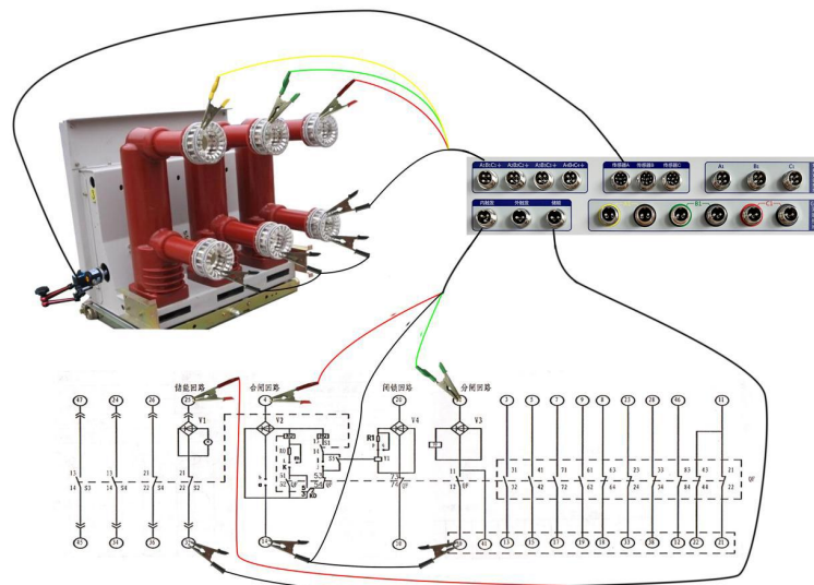
开关测试仪完整接线示意图
