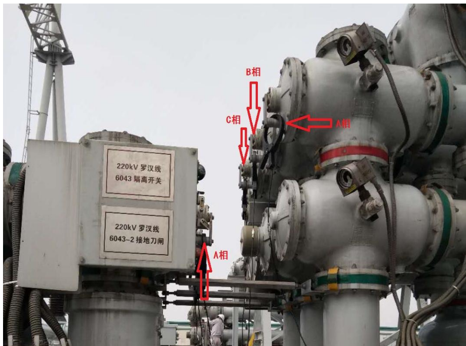
GIS 双端接地示意图：
