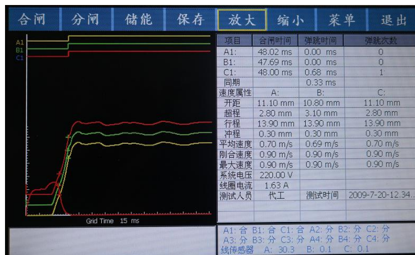
4、3路传感器合闸测试数据如下图：
