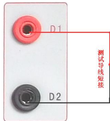
图 24，导线阻值清零接线图
