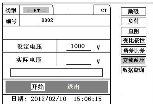
图 34, PT 交流耐压测试界面
