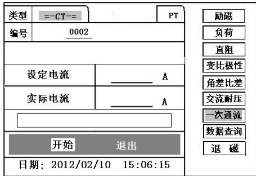
图 17、CT 一次通流测试界面
