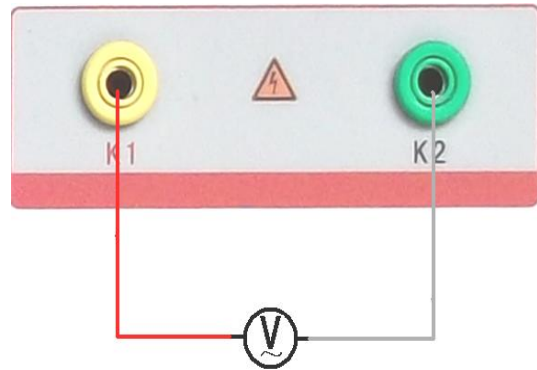
图 45, 电压校准接线
