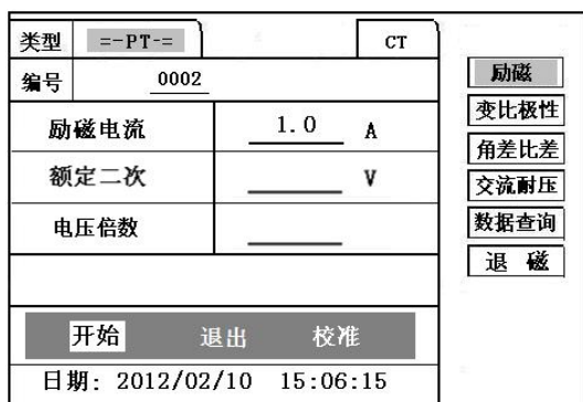
图 28, PT 励磁特性参数设置界面
